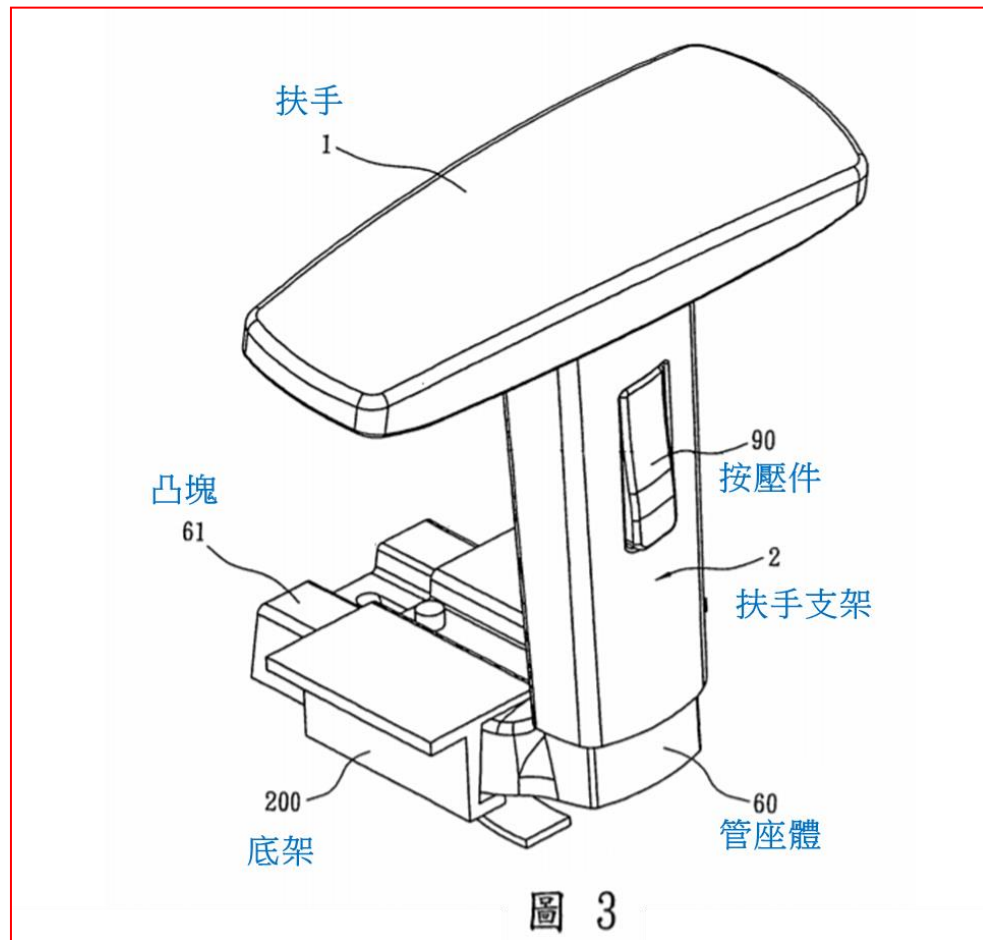
圖 3 係椅扶手高低調整裝置之立體圖
