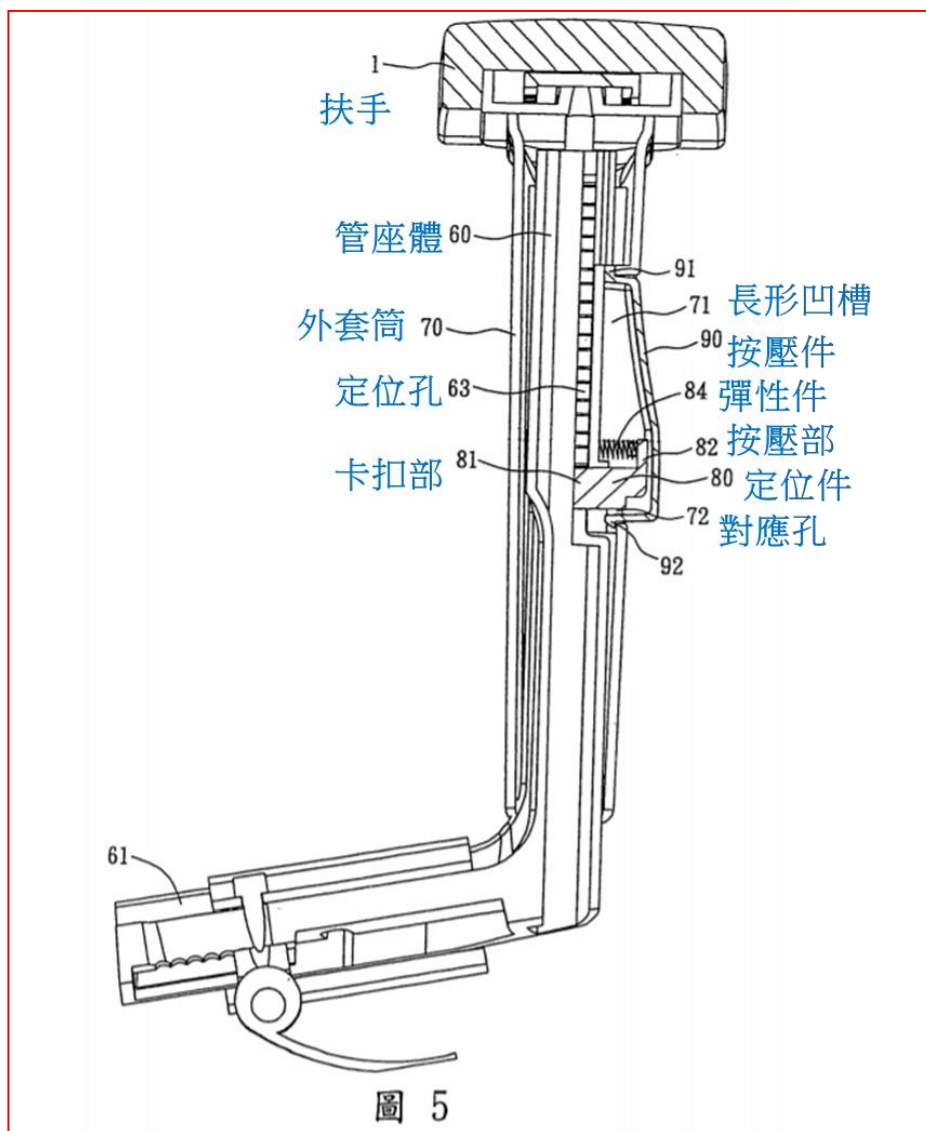
圖 5 係椅扶手高低調整裝置之使用狀態示意圖
