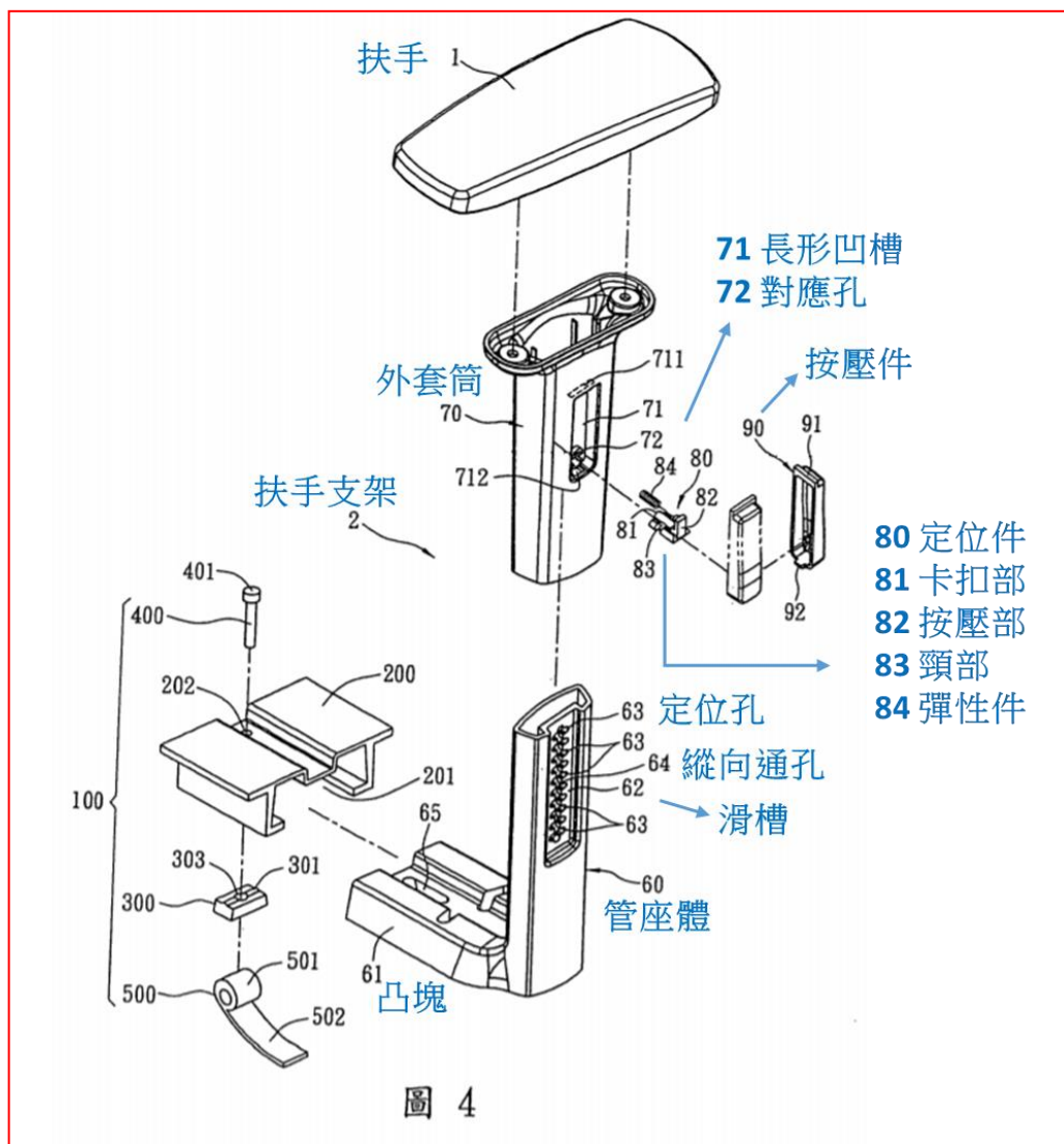
圖 4 係椅扶手高低調整裝置之分解圖
