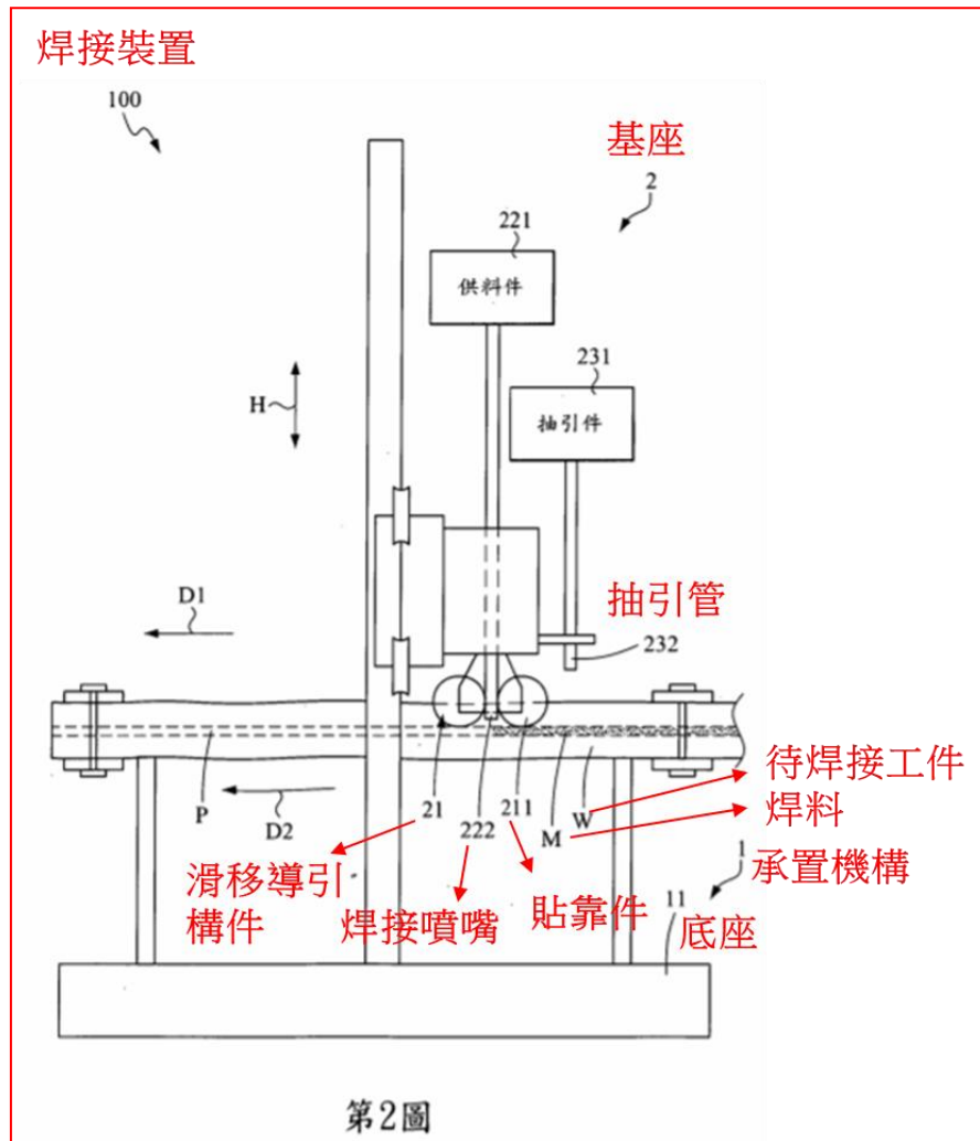
第 2 圖為顯示根據本創作的該實施例的焊接裝置的側視圖
