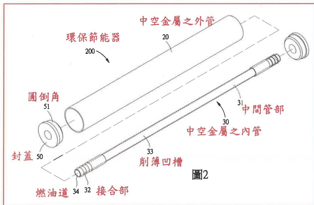
圖 2 為系爭專利實施例一立體分解圖。
