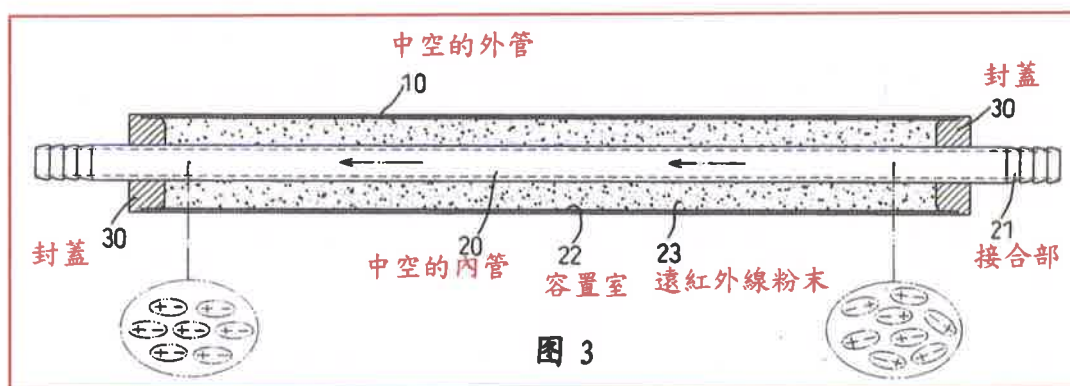
圖 3 為環保節能器之組合結構剖視圖。
