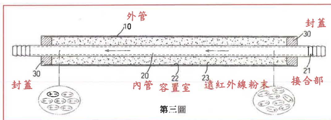
第三圖係鈦金環保節能器之組合剖視圖。
