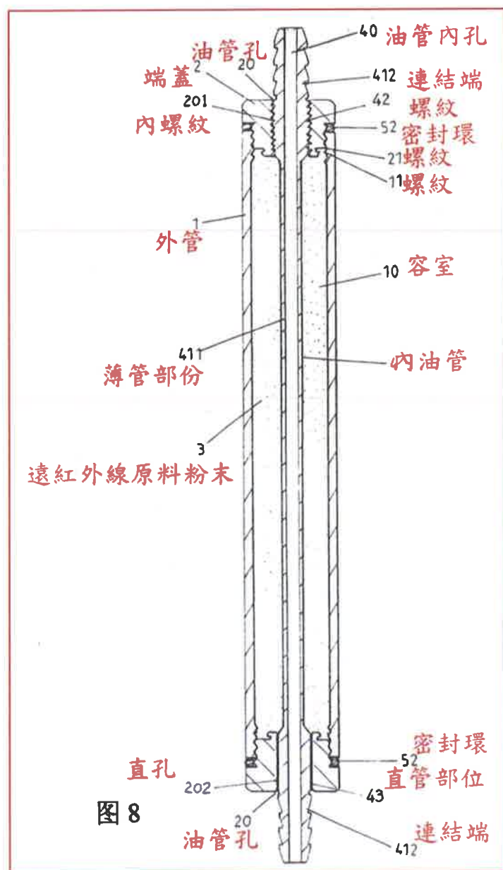
圖 8 係實施例結構示意圖。
