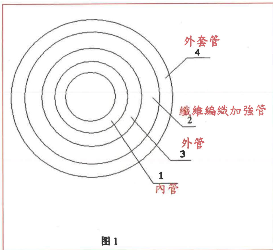
圖 1 為遠紅外燃油節能管的橫截面結構示意圖。
