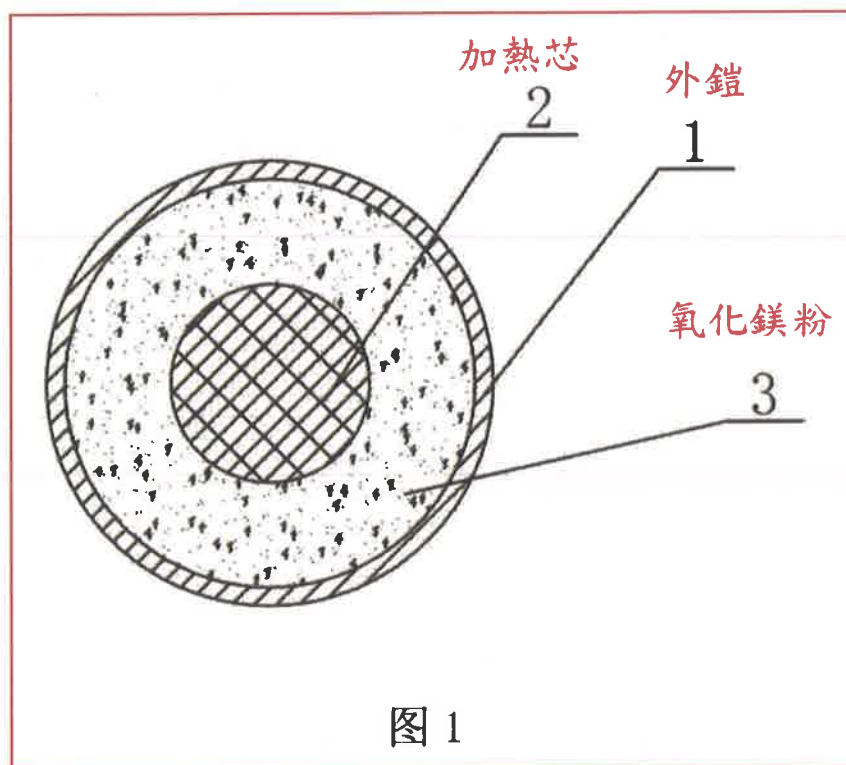
圖 1 為加熱管及加熱烘乾裝置之具體實施剖面圖。
