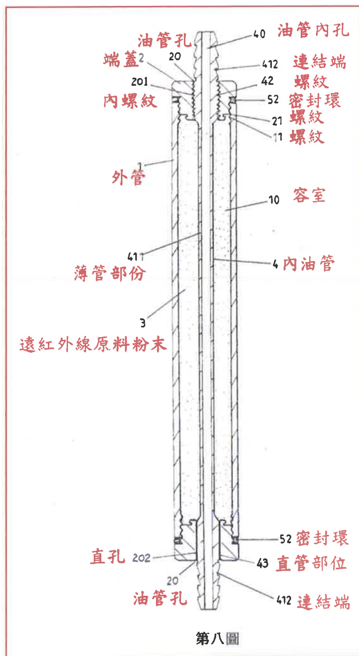
第八圖係省油加速器之實施例結構示意圖。
