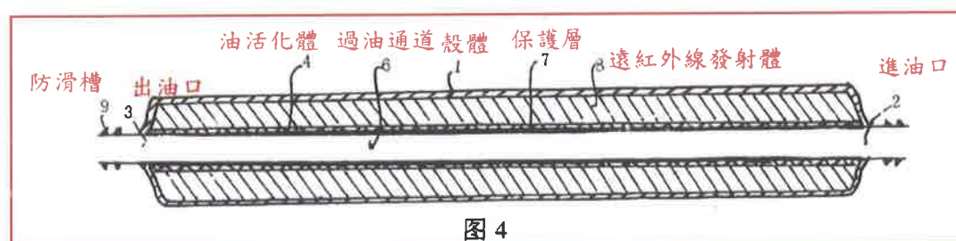
圖 4 為量子環保節油加速器之結構示意圖。
