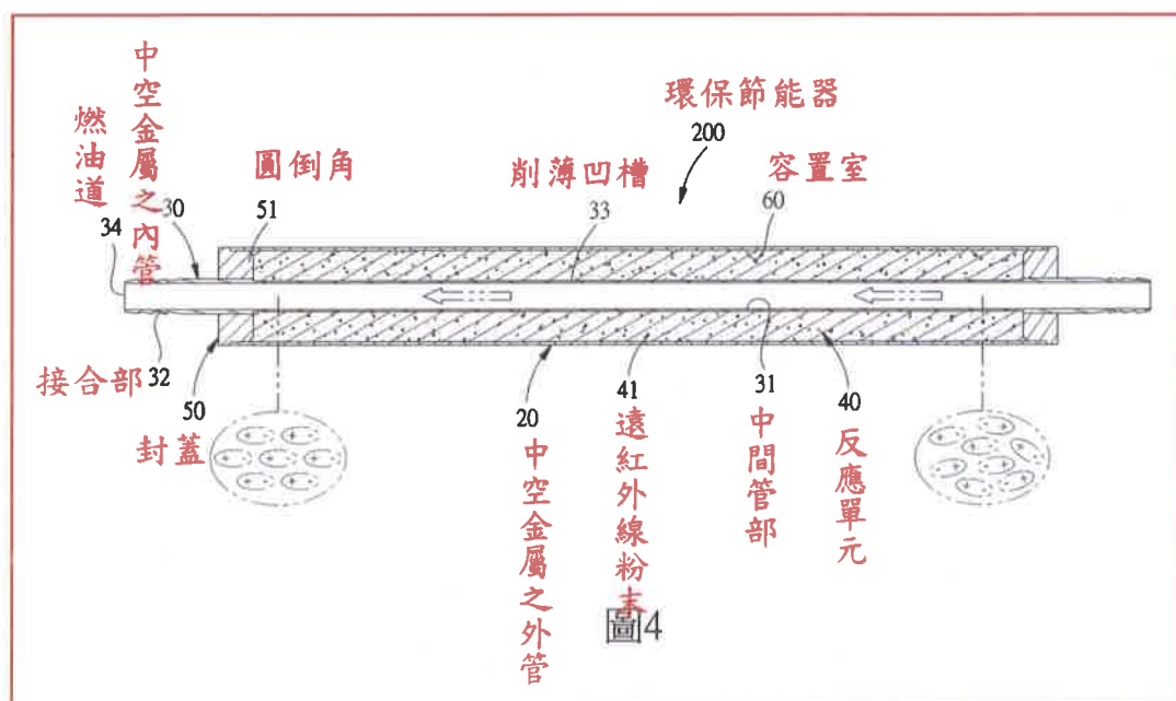
圖 4 為系爭專利實施例一使用剖面圖。
