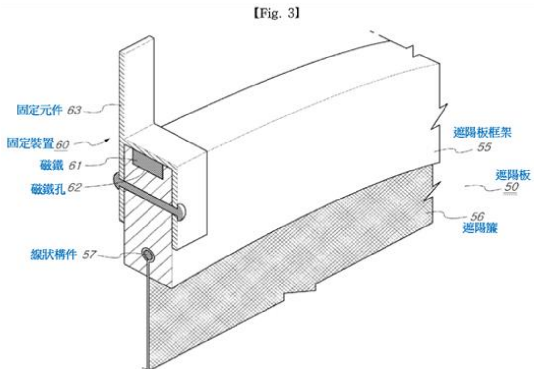
2.圖 3 為遮陽板 B 部分局部立體外觀圖
