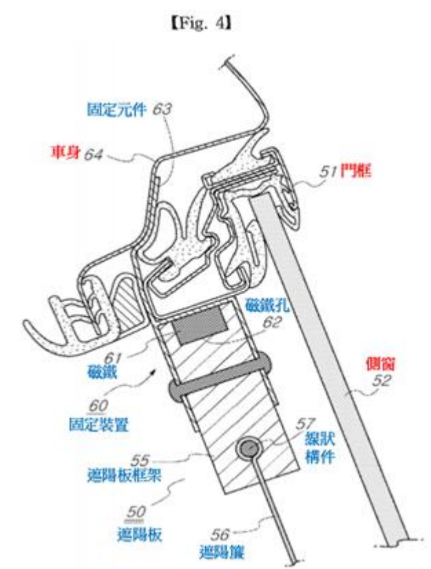
3.圖 4 為遮陽板 B 部分截面圖
