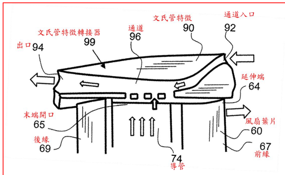
3. 圖 23 為冷卻風扇組件的截面圖
