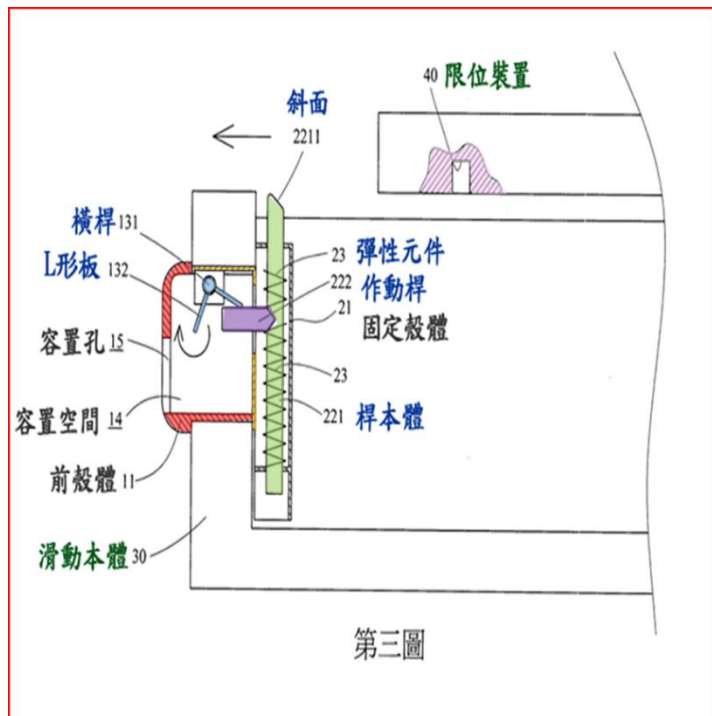
附圖 1-3：把手結構之開啟狀態剖視示意圖
