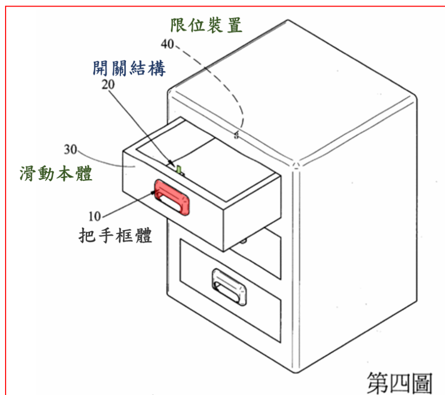
附圖 1-4：把手結構其一可行實施例之使用狀態示意圖
