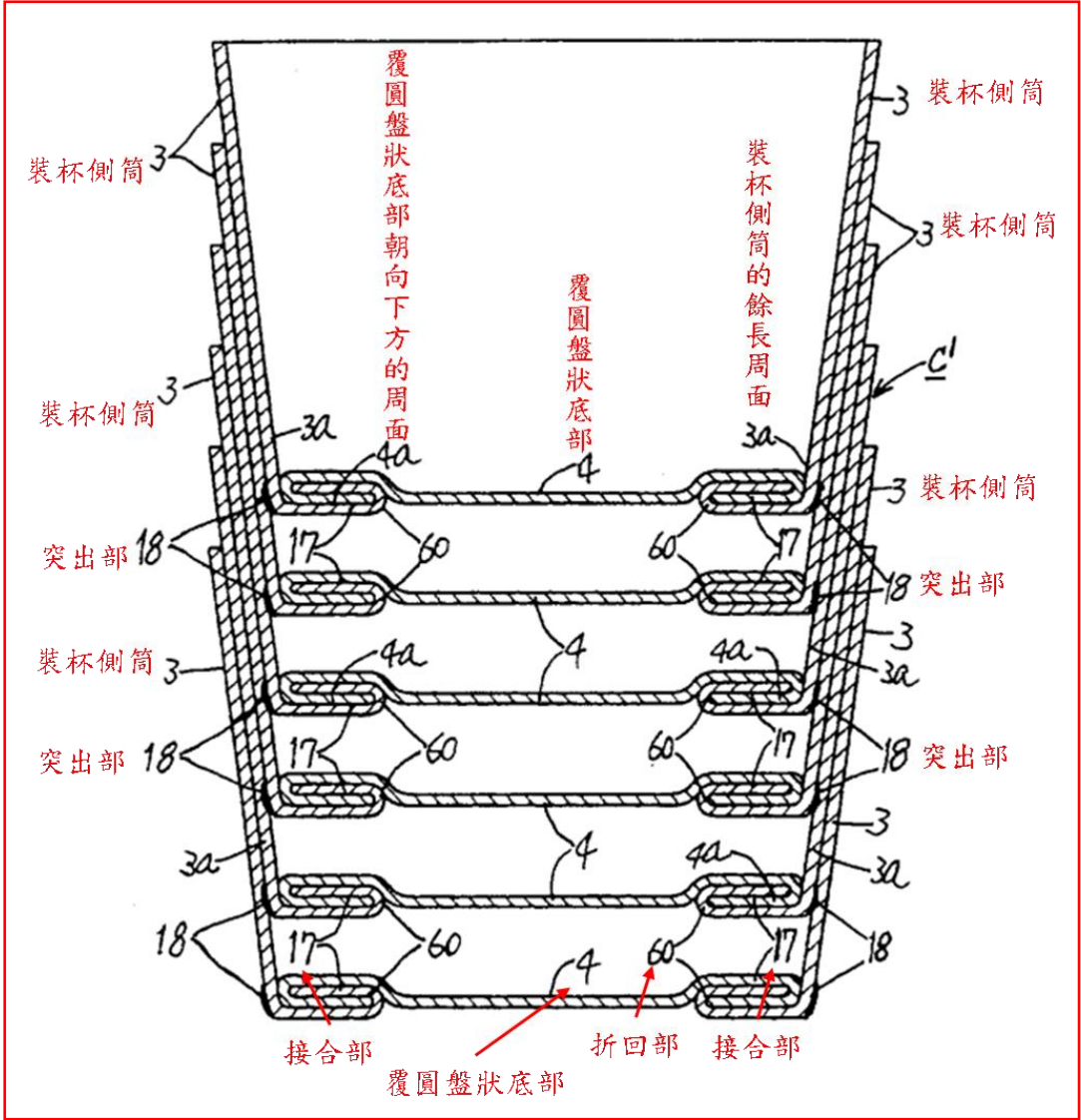
第 24 圖顯示將多數層傳統的紙製裝杯加以堆疊的例子的縱斷面
