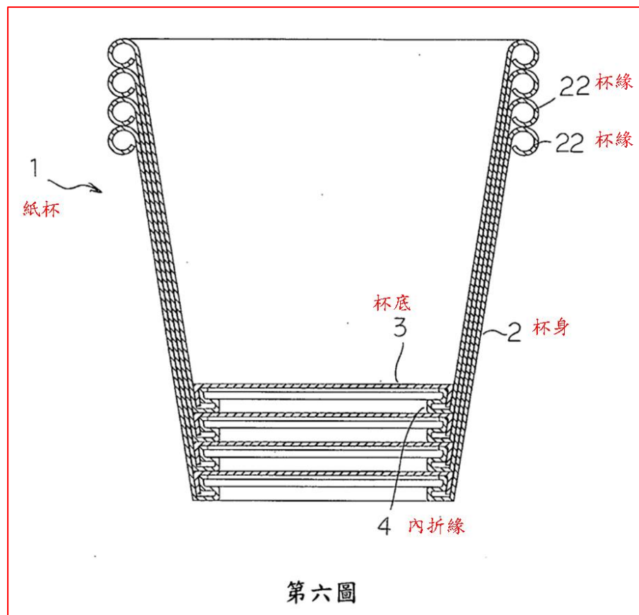
圖 6 為紙杯疊合圖
