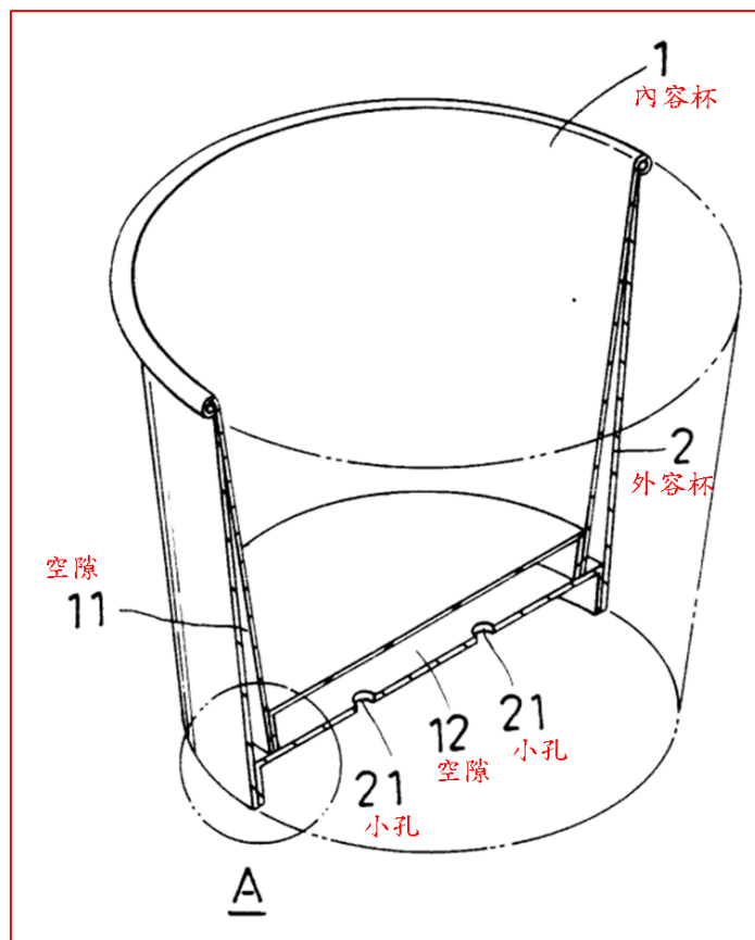
圖 1 為容器組剖面詳圖
