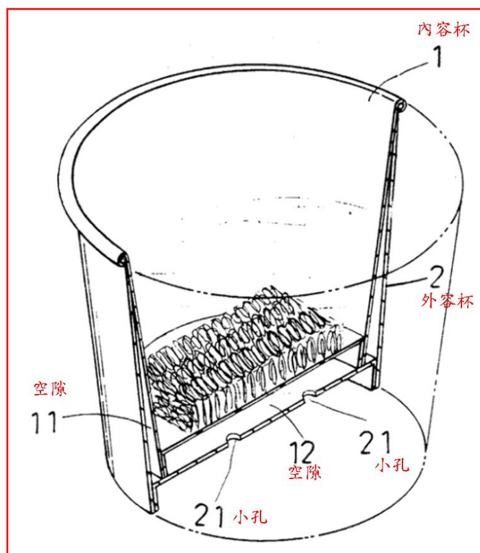
圖 2 為容器於裝盛滾沸熱開水進行速食食品沖泡的示意圖
