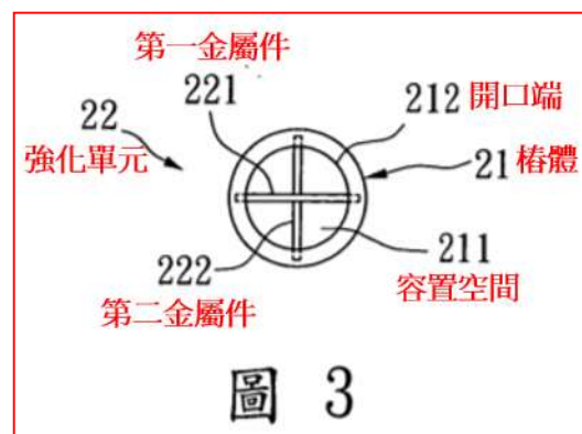
圖 3 圖 2 的俯視圖
