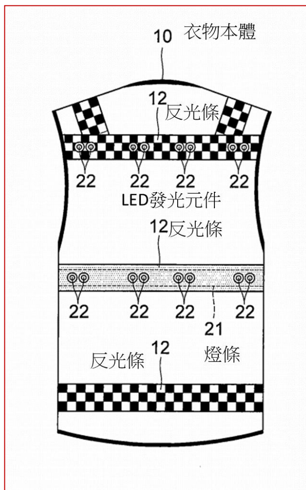
第 3 圖為本創作之後側構造示意圖
