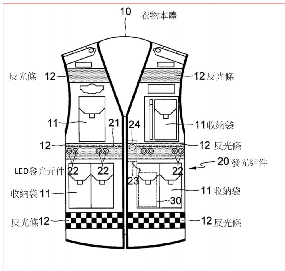
第 2 圖為本創作之前側構造示意圖
