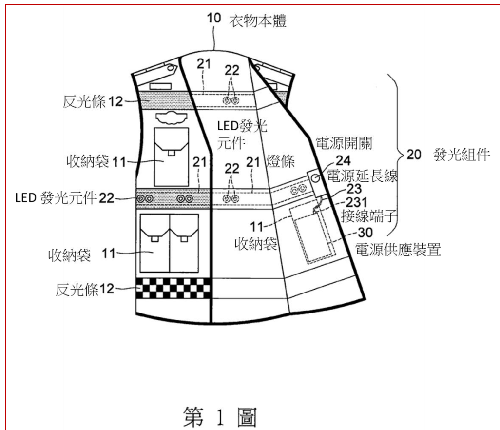
第 1 圖本創作之構造示意圖
