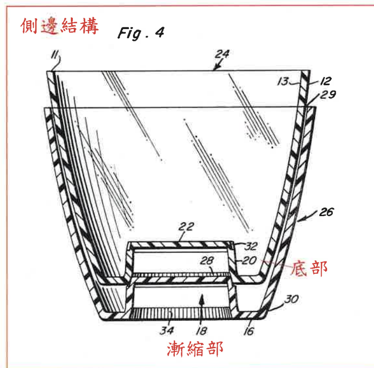
被證 2 圖 4 為杯體側視圖
