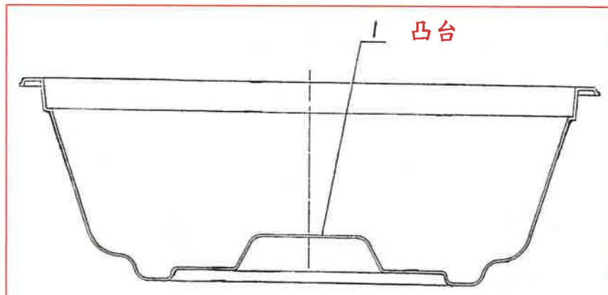
被證 4 圖 1 為紙漿模塑碗結構
