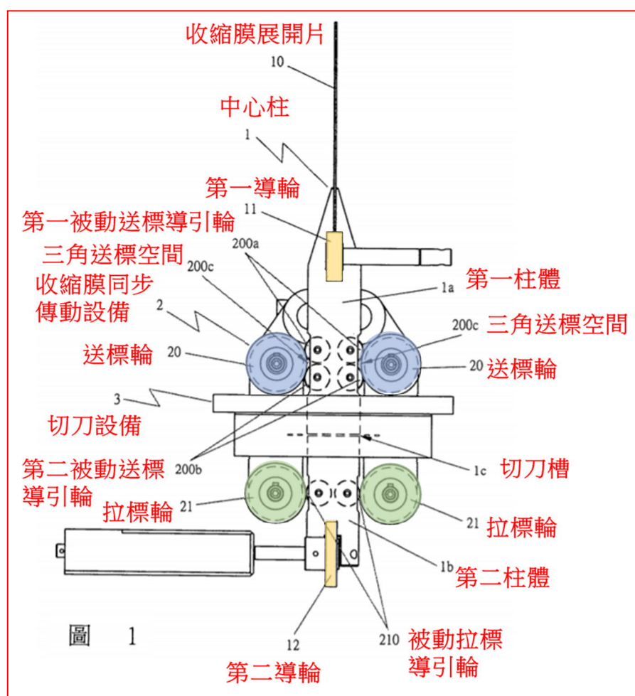
圖 1 為系爭專利套標機之部分前視圖。
