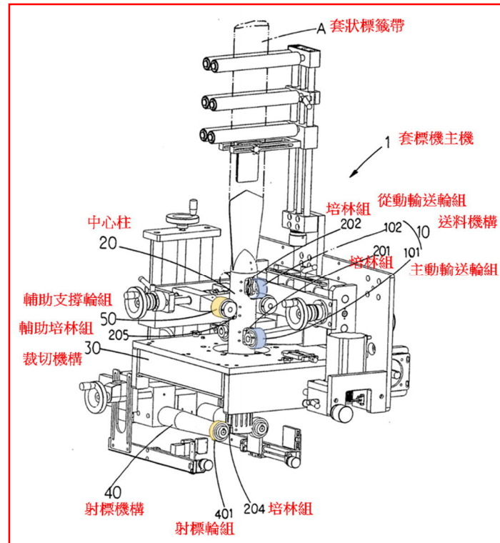
附圖三：被證 4 主要圖式
