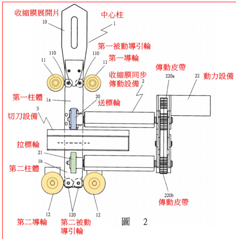
圖 2 為系爭專利套標機之部分側視圖。
