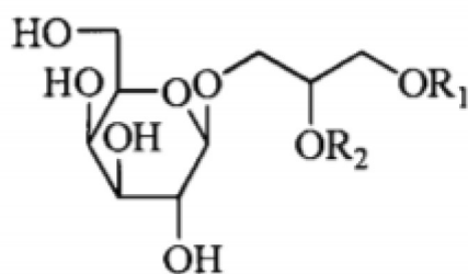
半乳糖脂化合物通式
