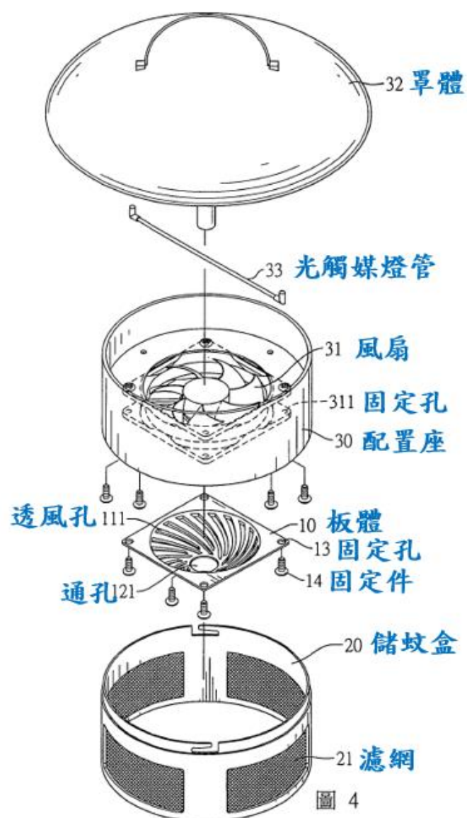
圖 4 係設置有系爭專利之捕蚊器分解圖
