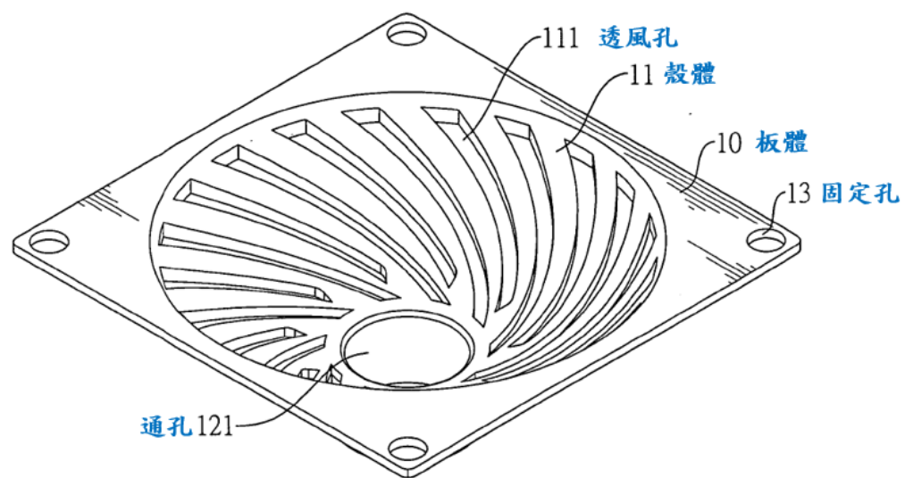
圖 1 係立體外觀圖
