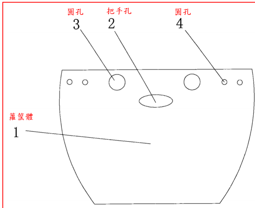
第十圖：正視圖和後視圖
