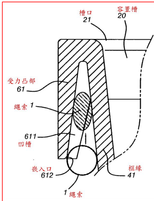
第六圖：系爭專利使用狀態剖示圖
