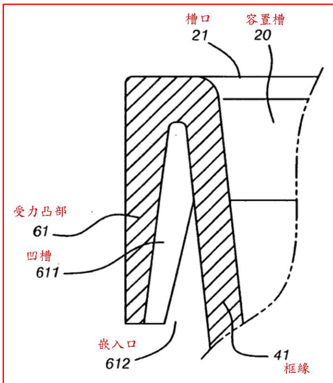
第五圖：第三圖之受力凸部的局部剖示圖
