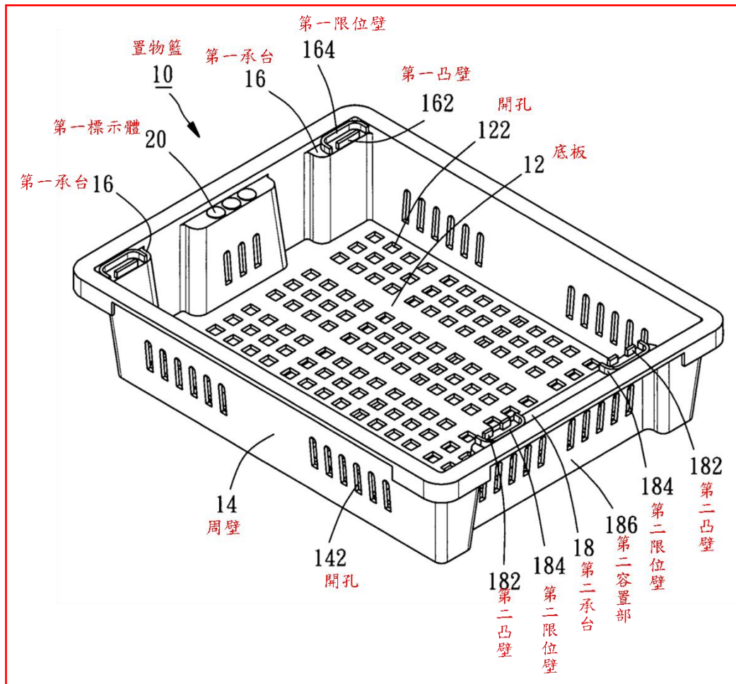
第十一圖：實施例之立體圖
