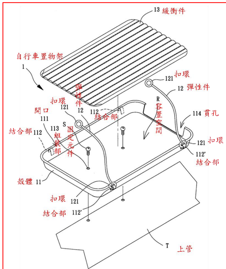
第八圖：第二實施例之立體分解圖
