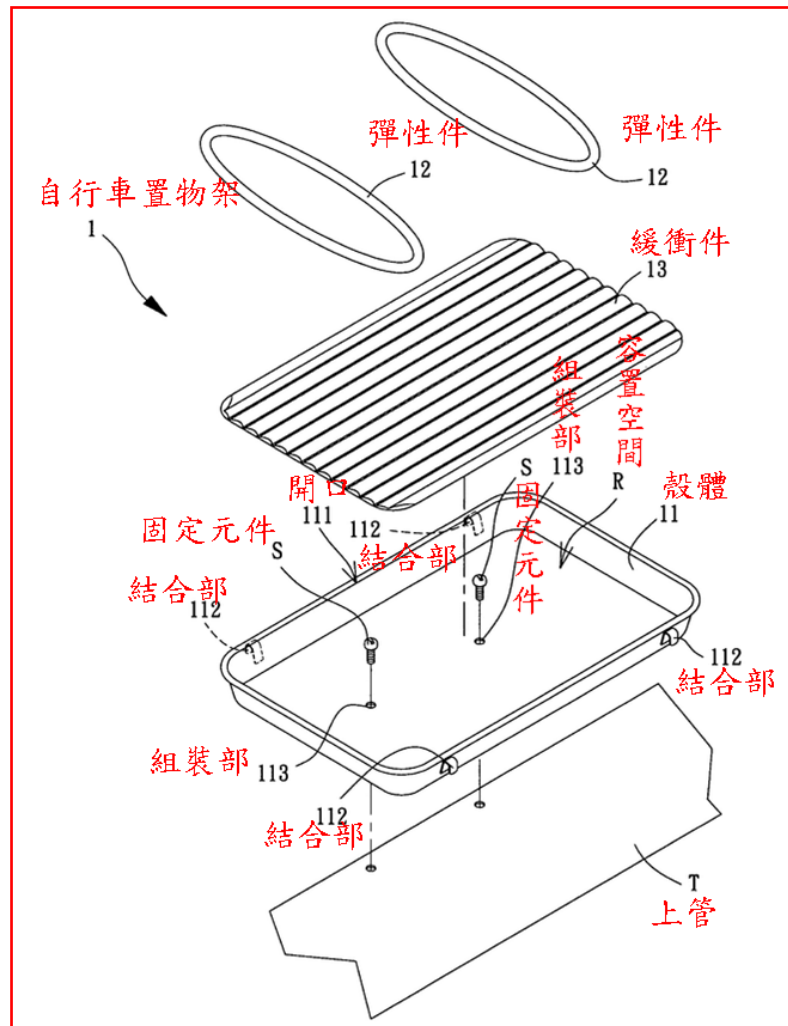
第七圖：第一實施例之立體分解圖
