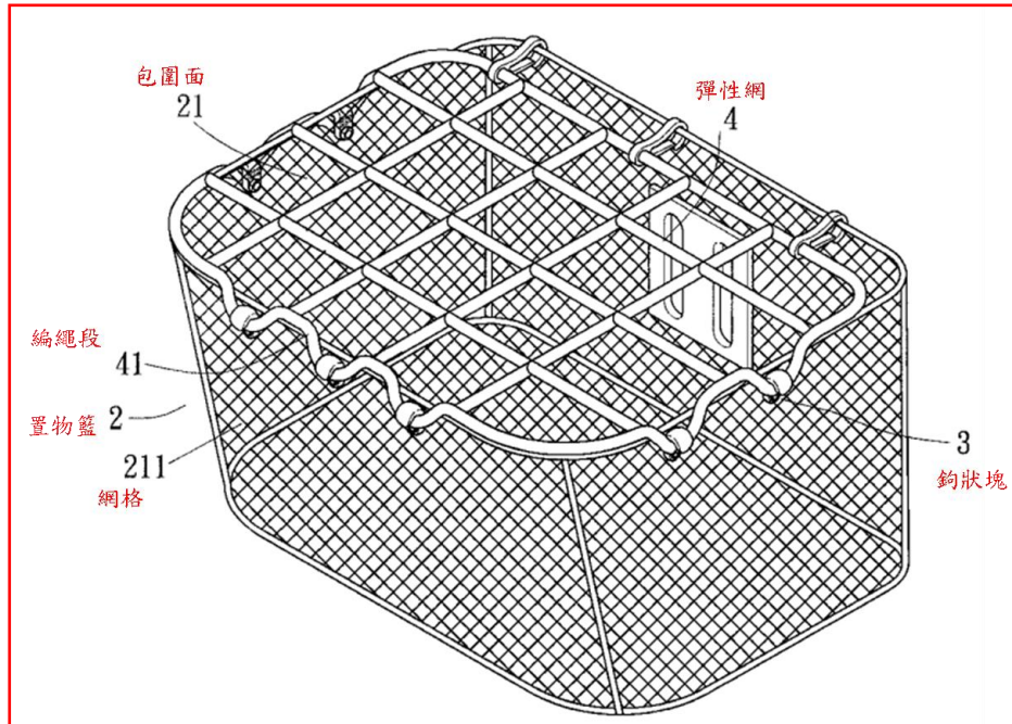
第十二圖：立體組合圖
