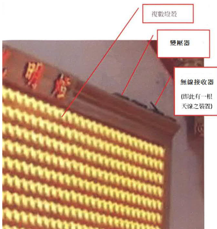
甲證 5-2 照片 I 局部放大圖之系爭產品之電壓器及無線接收器
