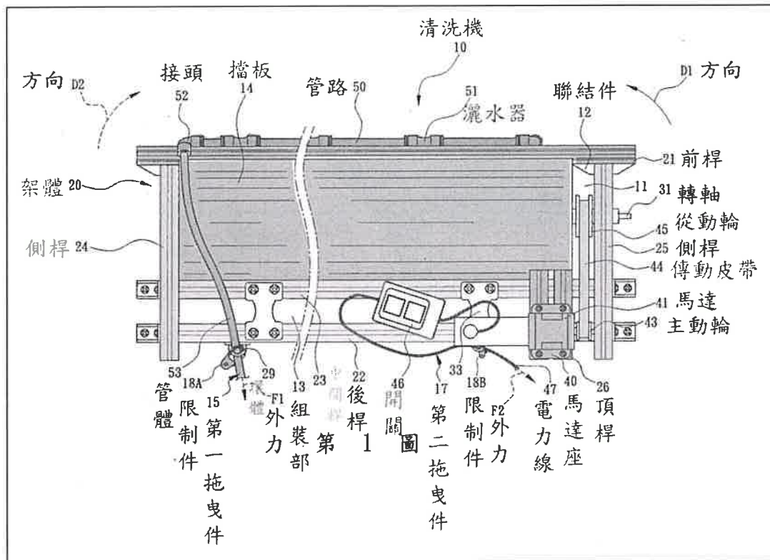
附圖二（系爭專利 2 主要圖式）：
