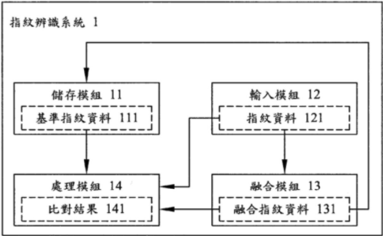
圖 1：系爭專利指紋辨識系統之方塊圖
