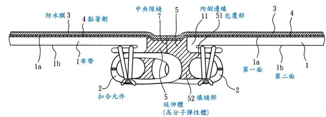
圖 5 為系爭專利 1 第三實施例之示意圖
