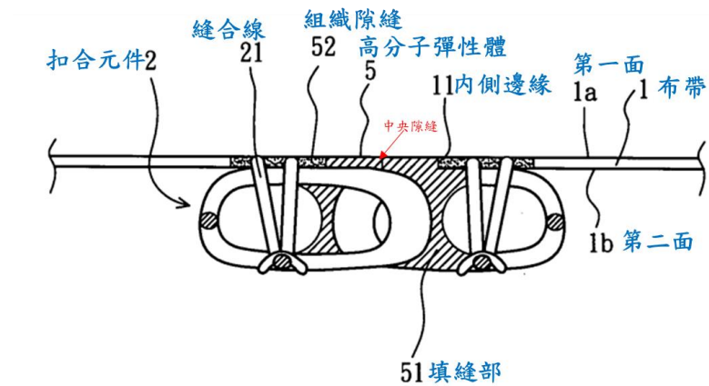
圖 1 為系爭專利 2 連續匝圈式 C 型拉鍊之防滲結構之各元件相對位置示意圖
