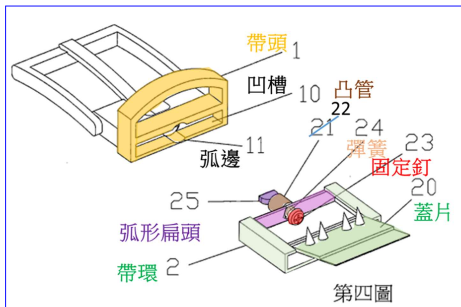
第 4 圖係第 3 圖帶頭和帶環部分組合示意圖。
