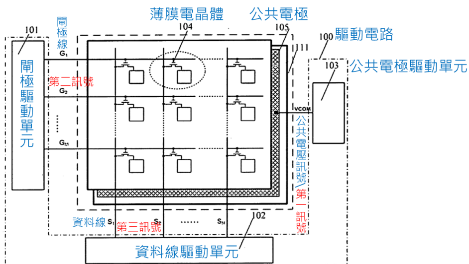
第5圖 系爭專利觸控顯示裝置一實施例之示意圖
