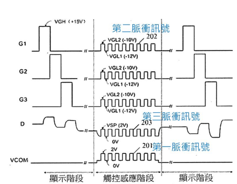
第6圖 圖5之觸控顯示裝置的驅動訊號的示意圖
