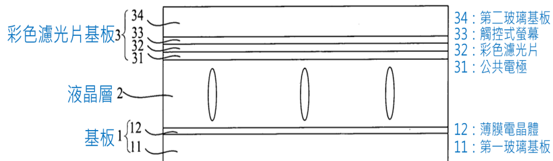
第1圖 習知一種內嵌式觸控式螢幕液晶顯示裝置的示意圖
