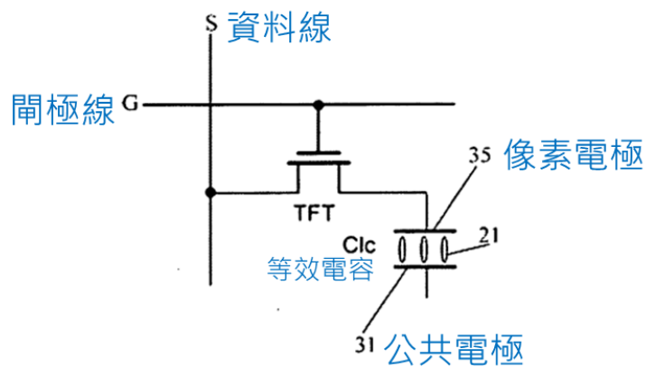
第2圖 圖1中一個子像素單元的等效電路圖
