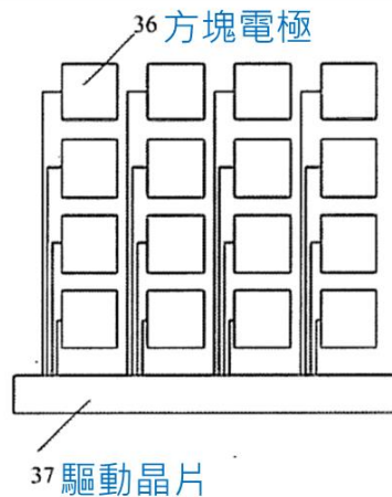
第3圖 習知一種兼具自電容觸控檢測功能的公共電極的示意圖
