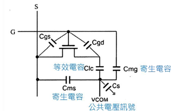
第4圖 習知公共電極用作觸控電極使一子像素單元的等效電路圖
