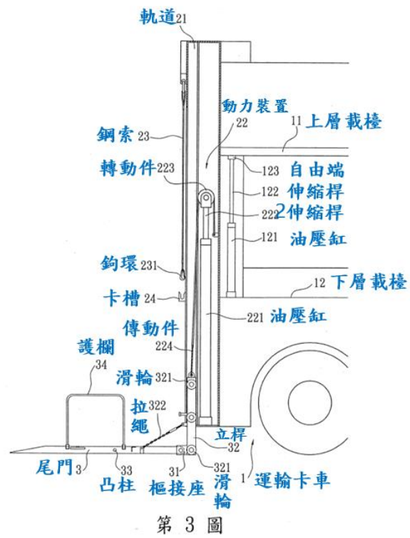
第 3 圖係尾門降至地面之示意圖
