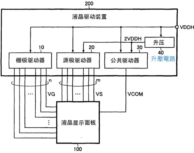
液晶显示装置之示意图
