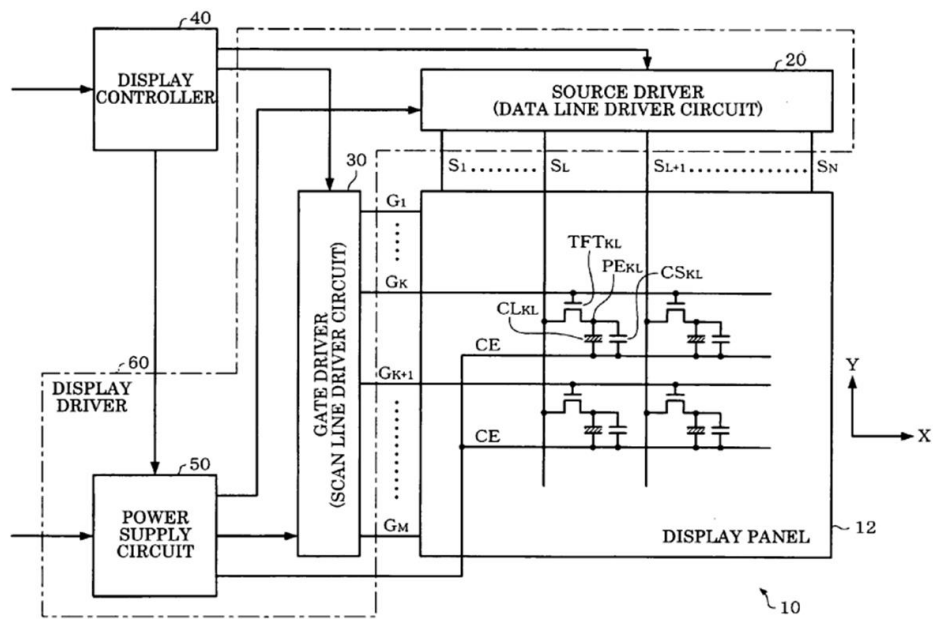
具電源供應電路之液晶裝置示意圖
