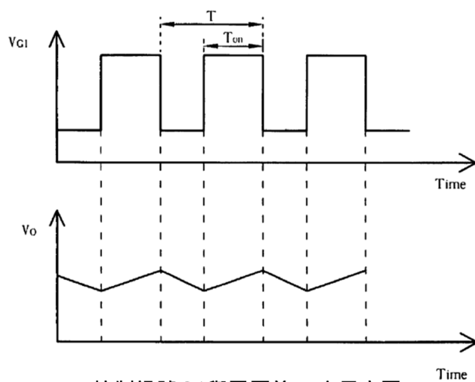
控制訊號G1與電壓差 V_o 之示意圖
