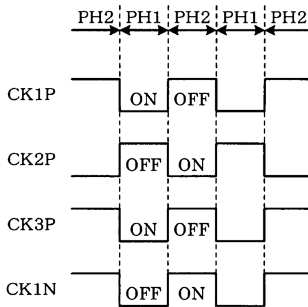
升壓電路各電晶體控制訊號之時序圖
