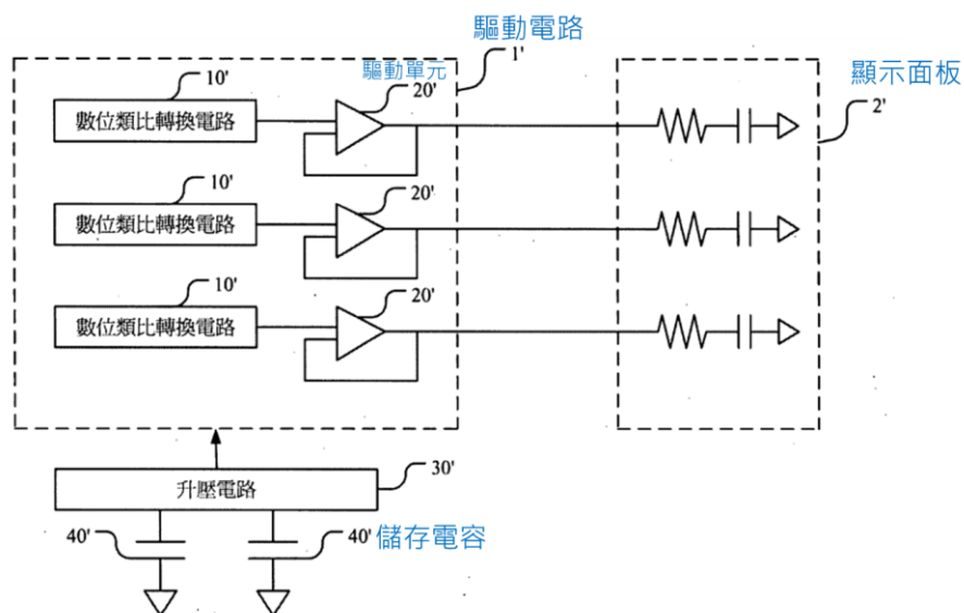
習知顯示面板之驅動電路
