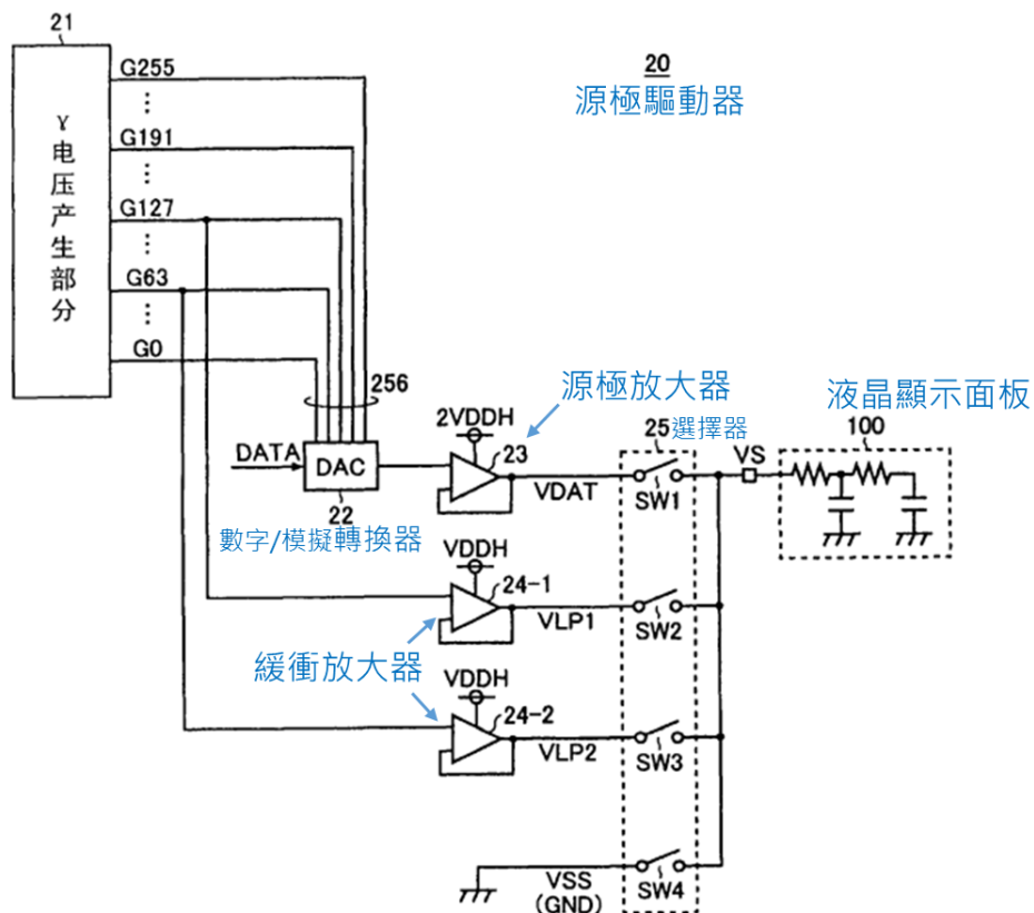
源極驅動器之配置電路示意圖
