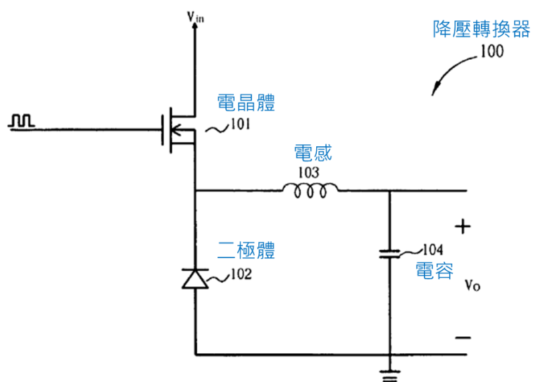
習知降壓轉換器之示意圖
