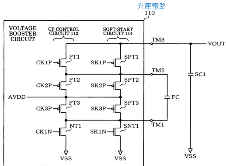
升壓電路之電路圖
