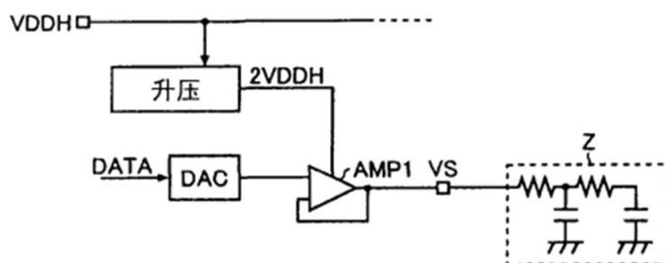
習知傳統源極驅動器之電路示意圖
