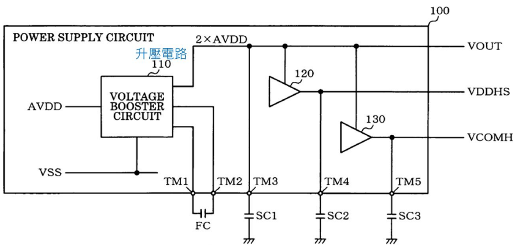
電源供應電路之電路圖
