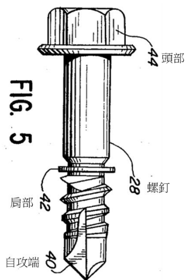
附圖 5：證據 5 之主要圖式
