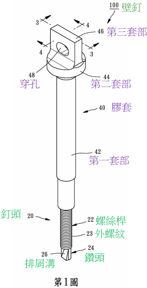
附圖 1：系爭專利主要圖式
