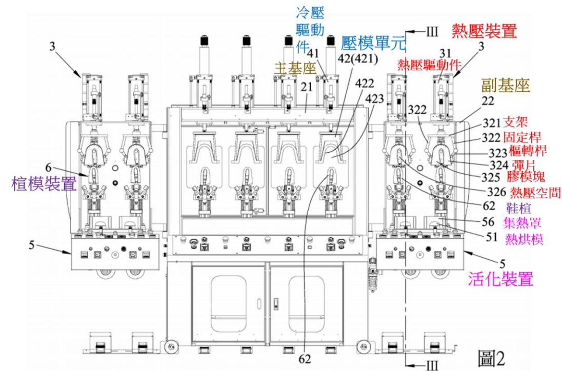
圖 2 是該實施例的一前視圖
