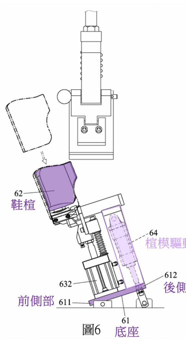
圖 6 是一不完整的側視圖，說明該實施例的其中一棺模單元地一底座在一裝設位置
