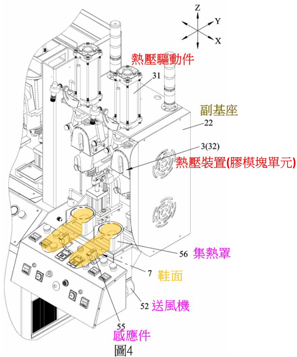
圖 4 是該實施例的一不完整的立體圖
