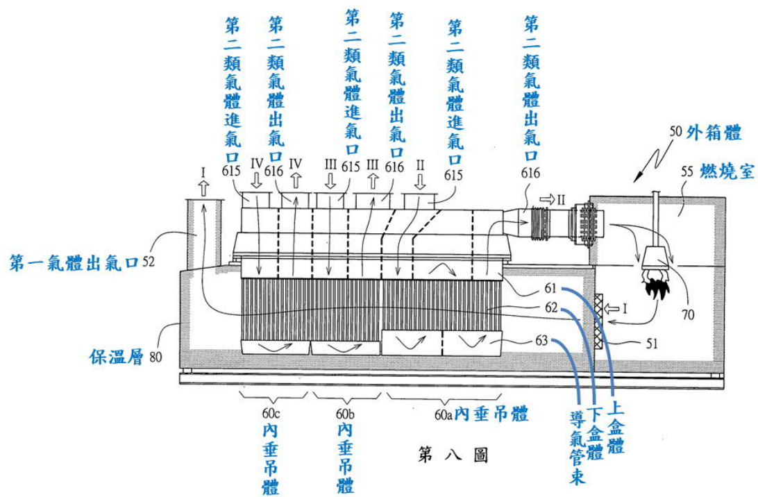
第八圖係焚化爐較佳實施例之結構說明圖。
