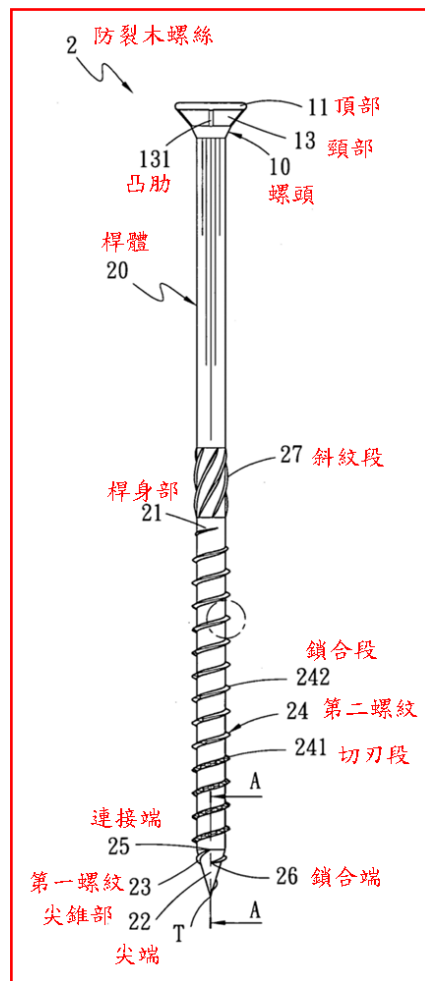
證據 4 第 3-1 圖為防裂木螺絲之平面示意圖。
