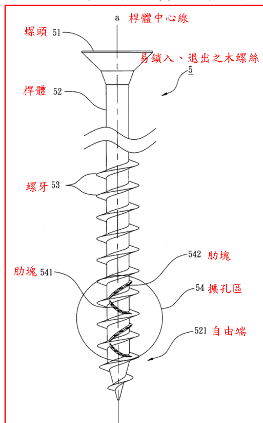
證據 2 圖 4 是木螺絲的第二較佳實施例之示意圖。
