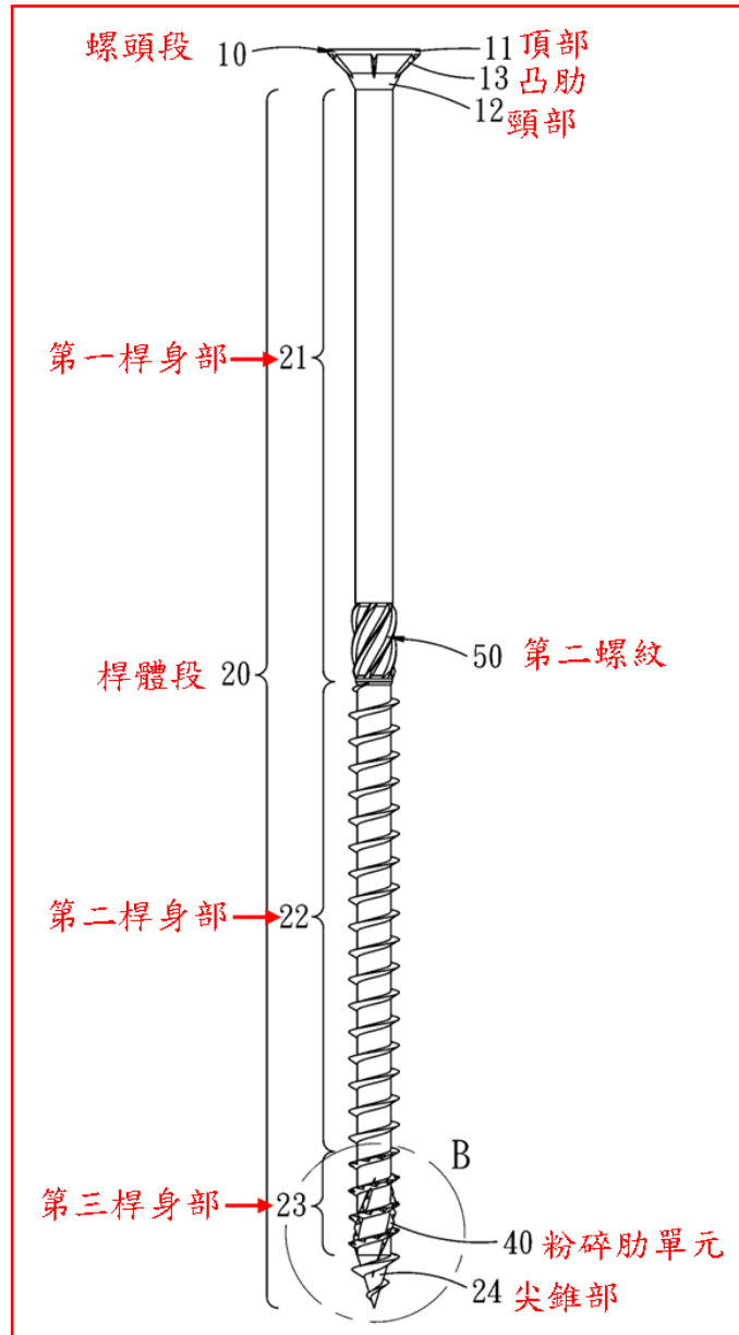
第 2-1 圖為系爭專利第一實施例之木螺絲結構之正視圖。
