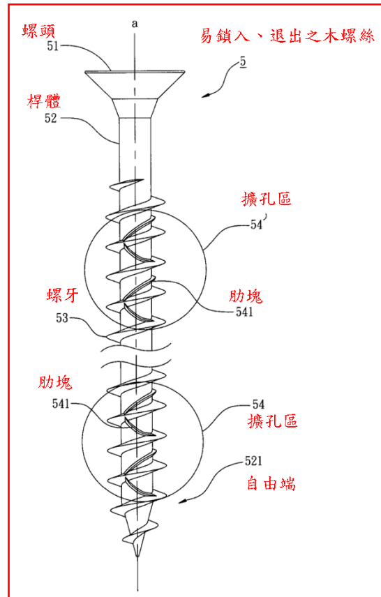
證據 2 圖 5 是木螺絲的第三較佳實施例。
