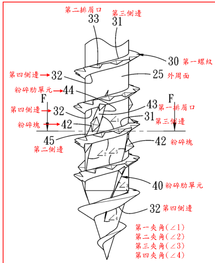
第 4-2 圖為系爭專利局部放大圖。
