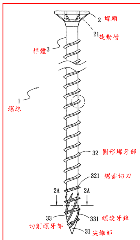
證據 3 第 2 圖為螺絲前視示意圖。
