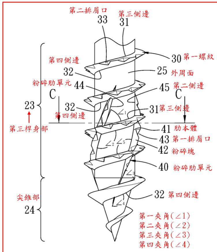
第 2-2 圖為系爭專利第 2-1 圖標示 B 之局部放大圖。
