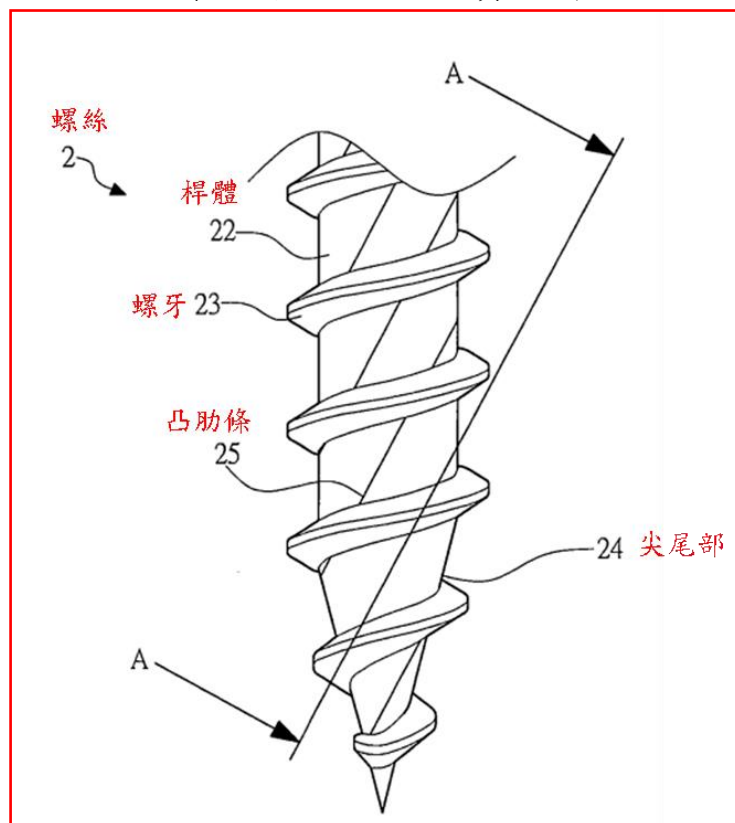
證據 5 圖七係圖六的局部放大圖。
