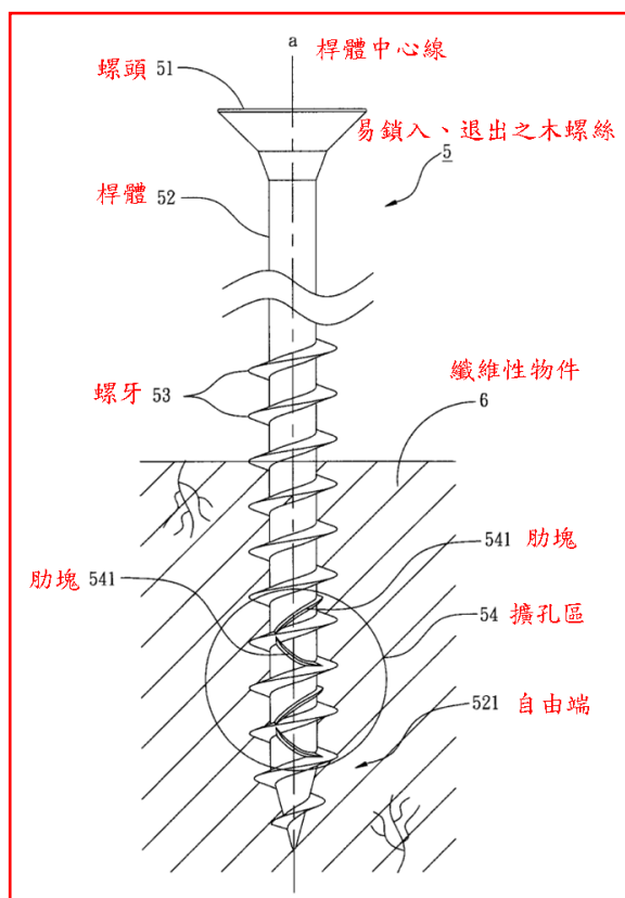
證據 2 圖 3 是木螺絲的第一較佳實施例之鎖合狀態示意圖。
