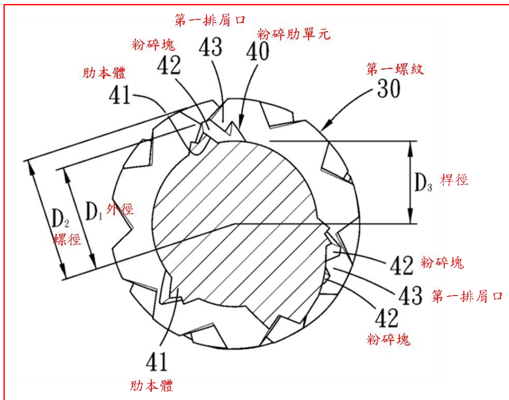
第 2-3 圖為系爭專利第 2-2 圖 C-C 剖線之剖面圖。
