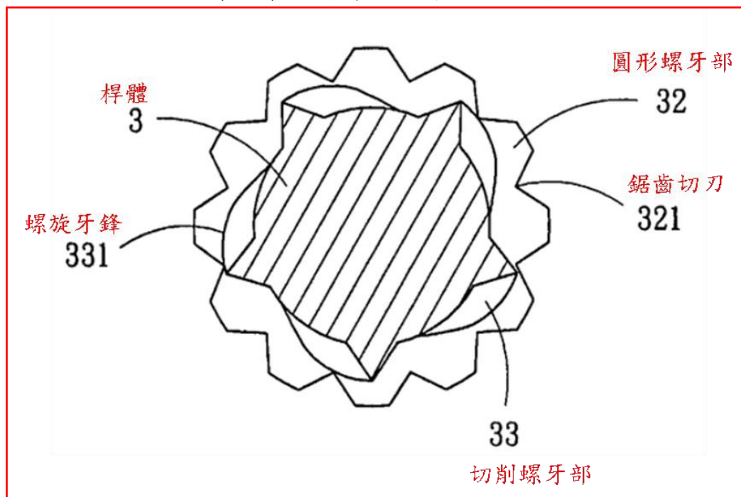
證據 3 第 3 圖係第 2 圖於 2A-2A 位置之剖面示意圖。
