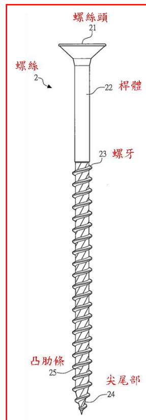
證據 5 圖六係螺絲之實施例。
