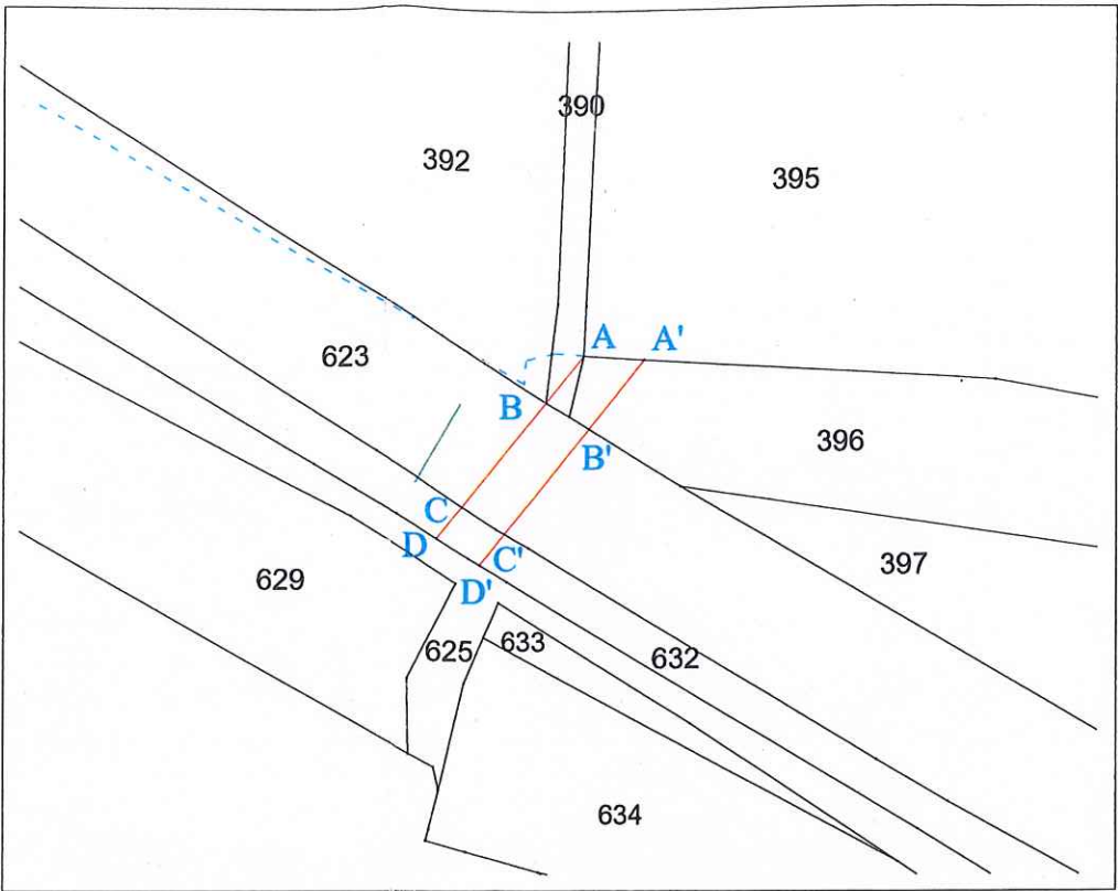
圖1 - 補充備位方案(路寬3米) 比例尺1/500
