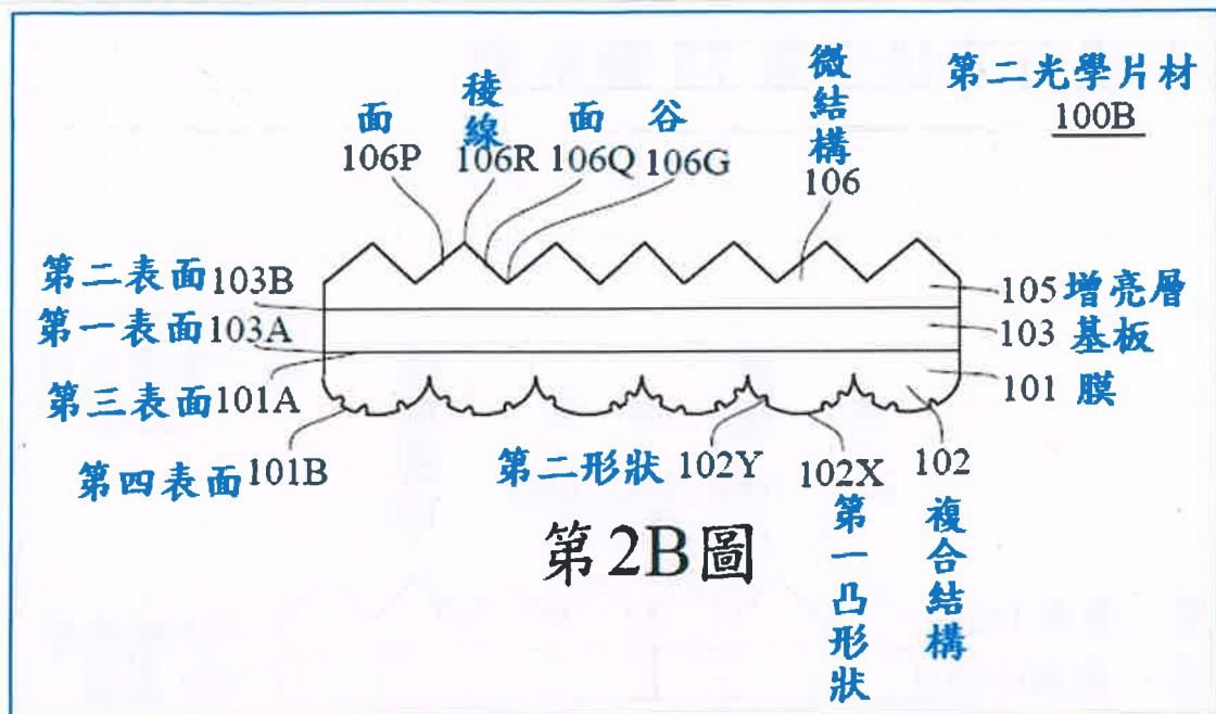
第 2A 至 2C 圖為系爭案第一、二、三光學片材剖面示意圖
