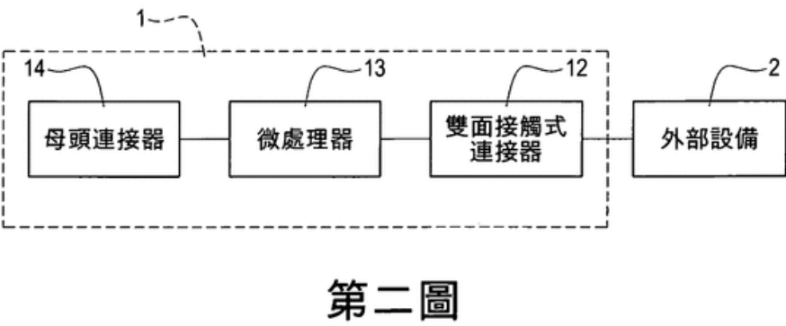
圖 4 (證據 2 第 2 圖)：證據 2 之第一具體實施例的電路方塊圖
