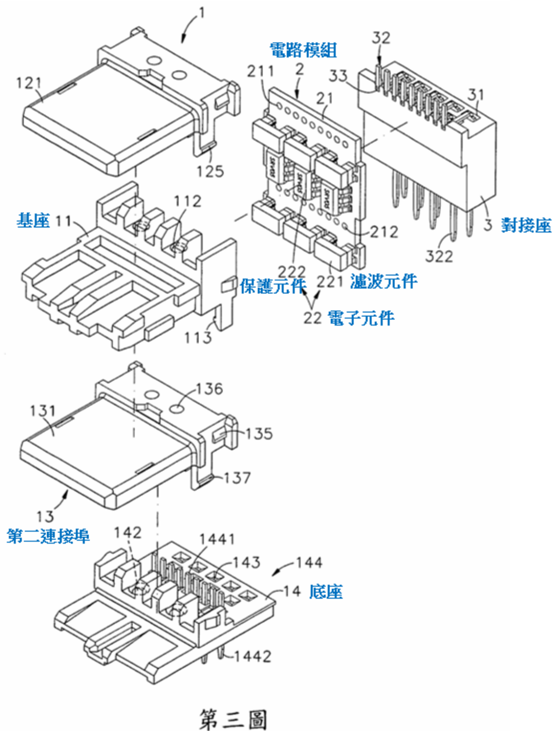
圖 10 (證據 6 第 3 圖)：證據 6 組裝時之立體分解圖(一)
