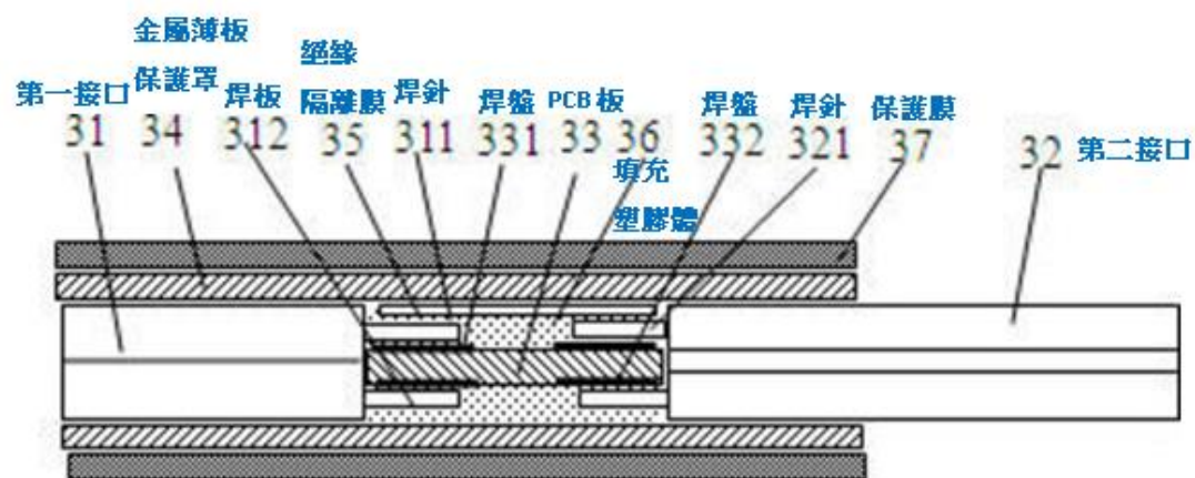
圖 9 (證據 5 第 5 圖)：證據 5 第二實施例的移動電源轉接頭的俯視結構示意圖
