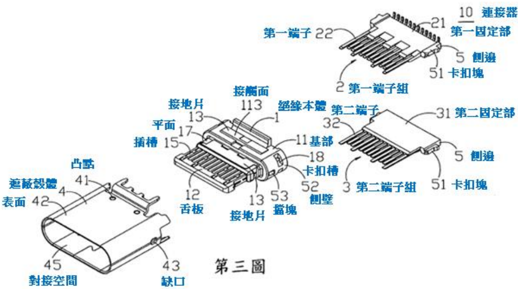
圖 8(證據 4 第 3 圖)：證據 4 第一實施例第一視角的立體分解圖
