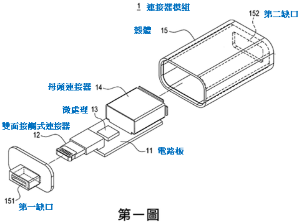
圖 3 (證據 2 第 1 圖)：證據 2 之第一具體實施例的立體分解圖
