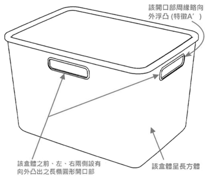
立體圖
