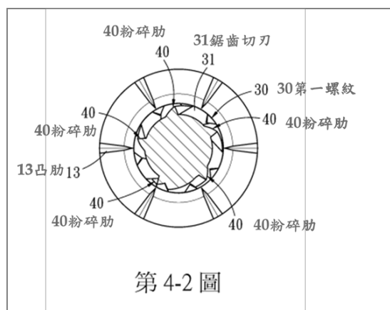
第 4-2 圖：為第 4-1 圖 B-B 剖線之剖面示意圖
