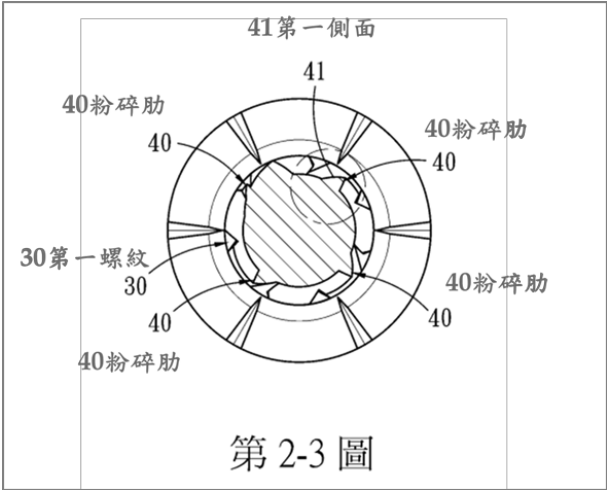
第 2-3 圖：為第 2-1 圖 A-A 剖線之剖面示意圖
