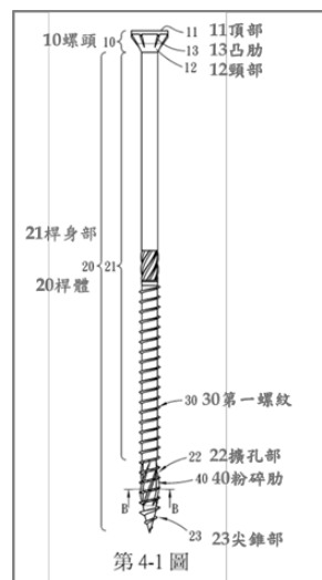
第 4-1 圖：為本發明低磨損螺絲結構之第二實施例之側面示意圖
