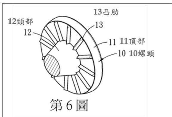
第 6 圖：為第 5-1 圖其螺頭之局部立體放大示意圖
