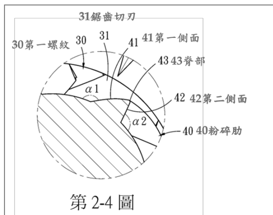
第 2-4 圖：為第 2-3 圖圈選處之局部放大圖
