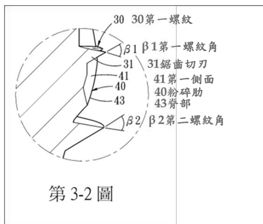
第 3-2 圖：為第 3-1 圖圈選處之局部放大圖
