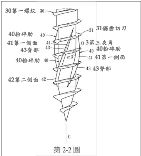
第 2-2 圖：為第 2-1 圖圈選處之局部放大圖
