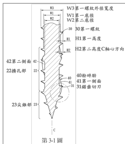
第 3-1 圖：為第 2-1 圖圈選處之剖面示意圖
