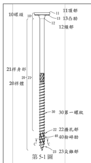
第 5-1 圖：為本發明低磨損螺絲結構之第三實施例之側面示意圖
