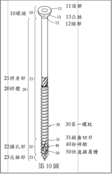
第 10 圖：為本發明低磨損螺絲結構之第七實施例之立體示意圖
