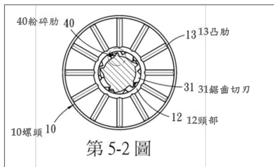
第 5-2 圖：為第 5-1 圖 C-C 剖線之剖面示意圖
