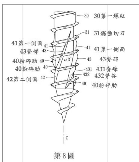
第 8 圖：為本發明低磨損螺絲結構之第五實施例之桿體局部側面示意圖
