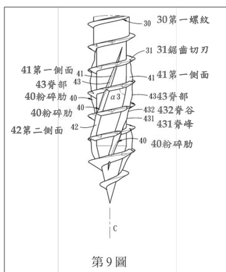
第 9 圖：為本發明低磨損螺絲結構之第六實施例之桿體局部側面示意圖
