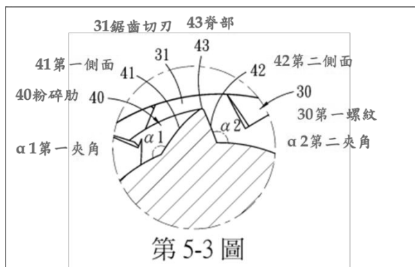
第 5-3 圖：為第 5-2 圖圈選處之放大示意圖
