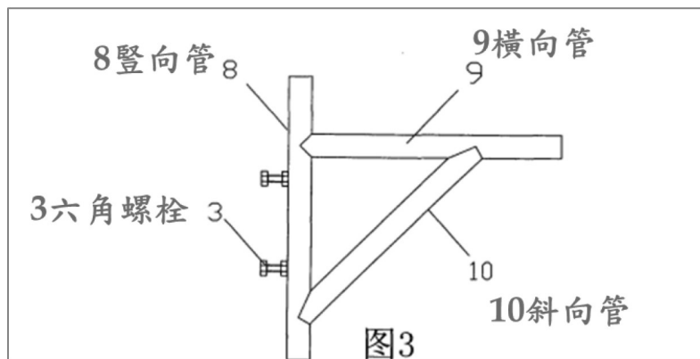
圖 3 為管式三角撐 2 的結構示意圖
