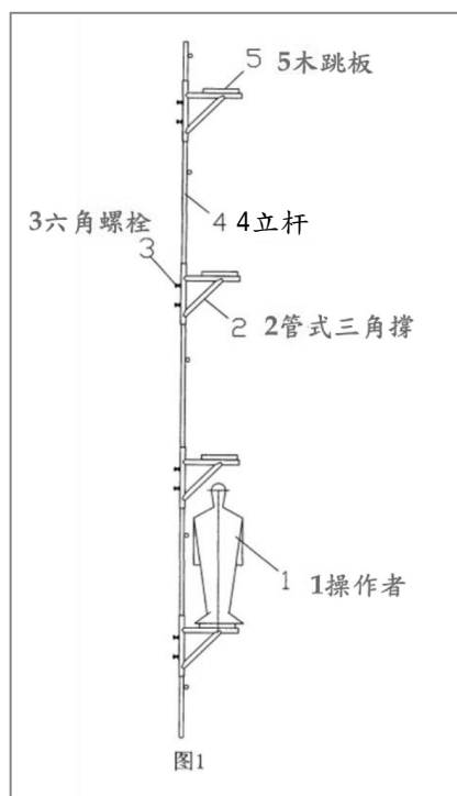
圖 1 為單組多層狀操作架的側視圖
