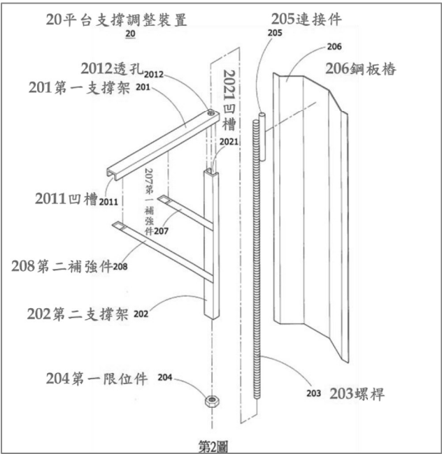
第 2 圖為系爭專利之結構組成示意圖
