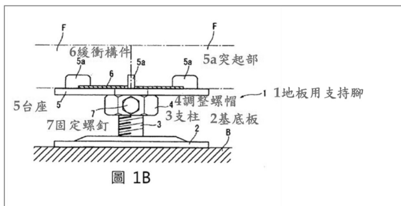
圖 1B 為實施形態之地板用支持腳正視圖
