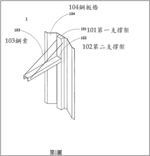
第 1 圖為一種習知的平台支撐裝置
