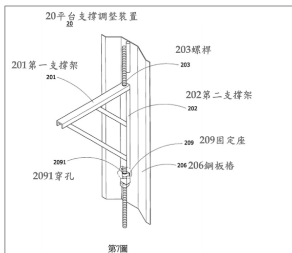
第 7 圖為系爭專利之另一實施例(二)
