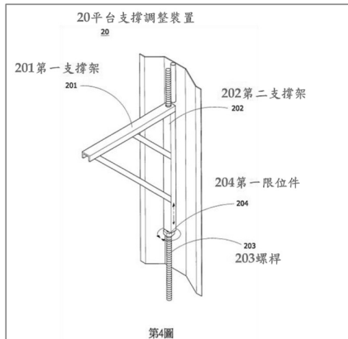
第 4 圖為系爭專利之實施示意圖(一)
