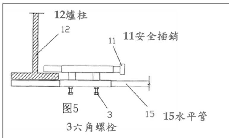
圖 5 為管式安全銷的使用狀態圖
