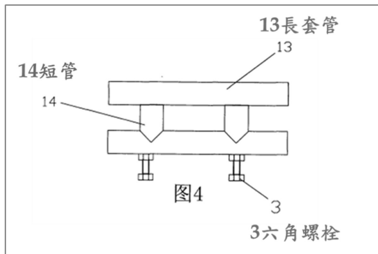
圖 4 為管式安全銷的結構示意圖
