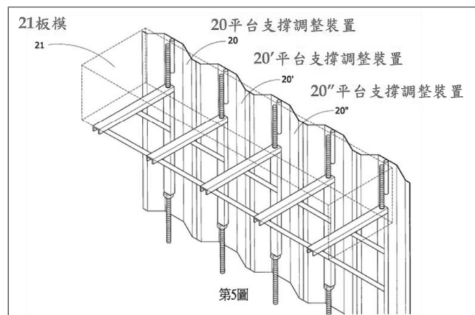
第 5 圖為系爭專利之實施示意圖(二)
