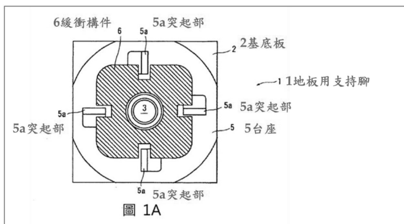
圖 1A 為實施形態之地板用支持腳俯視圖
