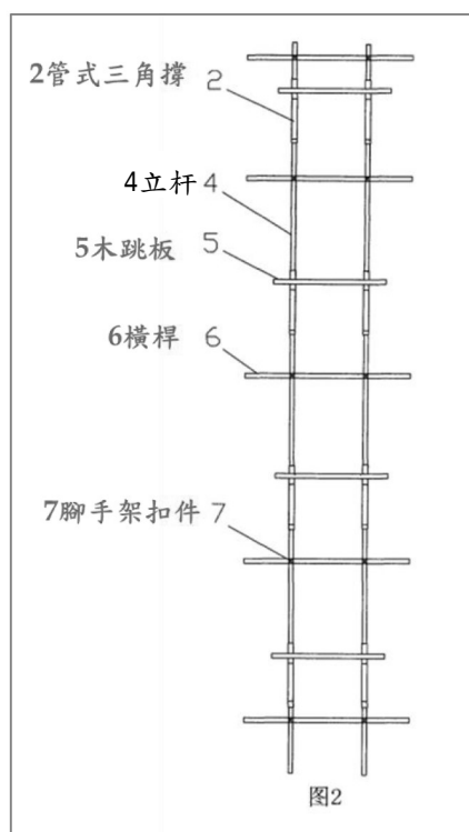
圖 2 為單組多層狀操作架的平視圖
