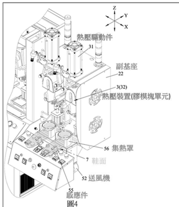
圖 4 是該實施例的一不完整的立體圖
