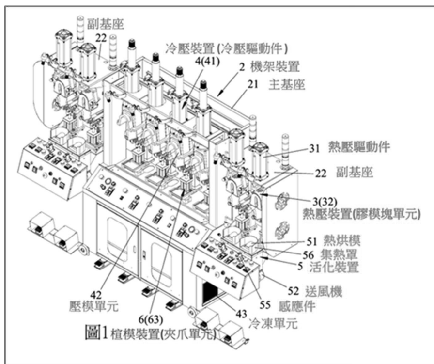
圖 1 是具有活化裝置的後踵定型機的一實施例的一立體圖
