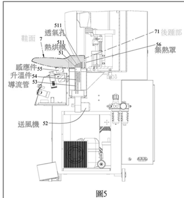
圖 5 是一不完整的剖視圖，說明該實施例的一熱烘模供一鞋面套設的狀態
