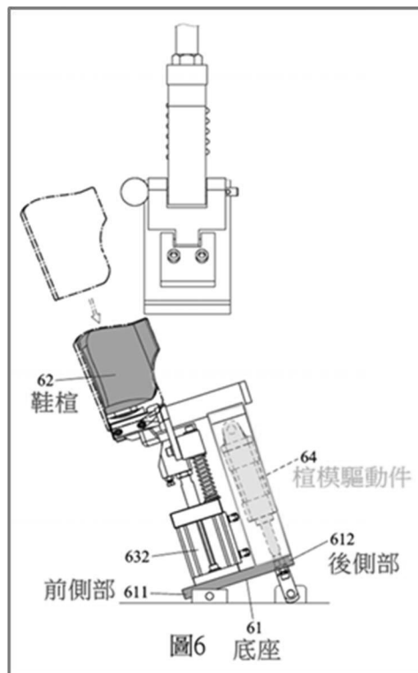
圖 6 是一不完整的側視圖，說明該實施例的其中一楦模單元地一底座在一裝設位置
