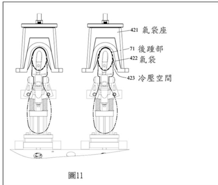
圖 11 是一不完整的前視圖，說明該等氣袋在一充氣狀態
