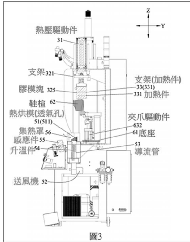
圖 3 是沿圖 2 中的線Ⅲ-Ⅲ所取得的一剖視圖
